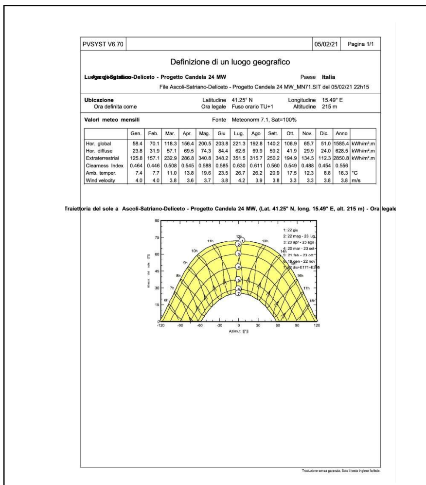
Figura 16-2 Calcolo dell'irraggiamento solare PVsyst-dati METEONORM 7.1
