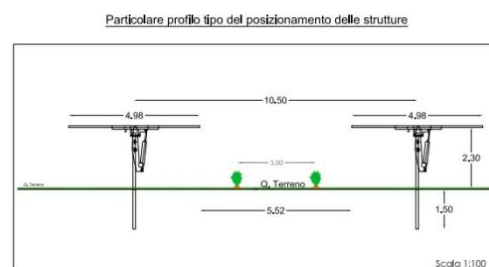
Figura 15-1 predisposizione pannelli Campo 1-2
