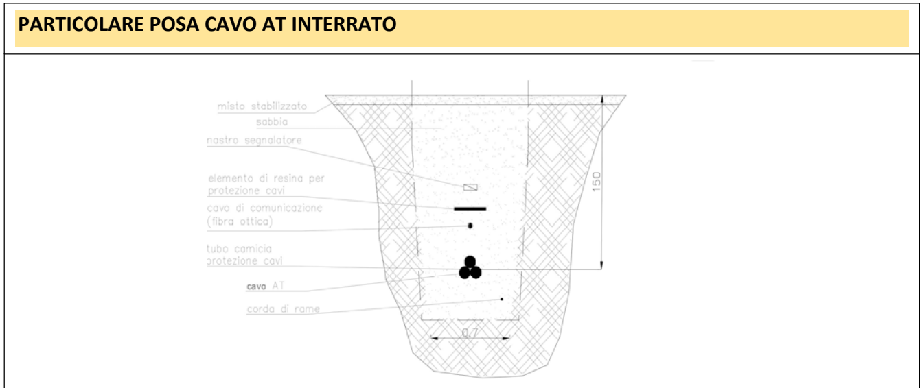
Figura 9-1 Particolare Posa Cavo AT Interrato
