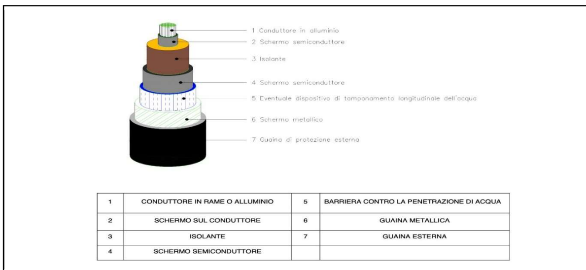
Figura 7-1 Caratteristiche tecniche Cavo AT per trasporto energia
