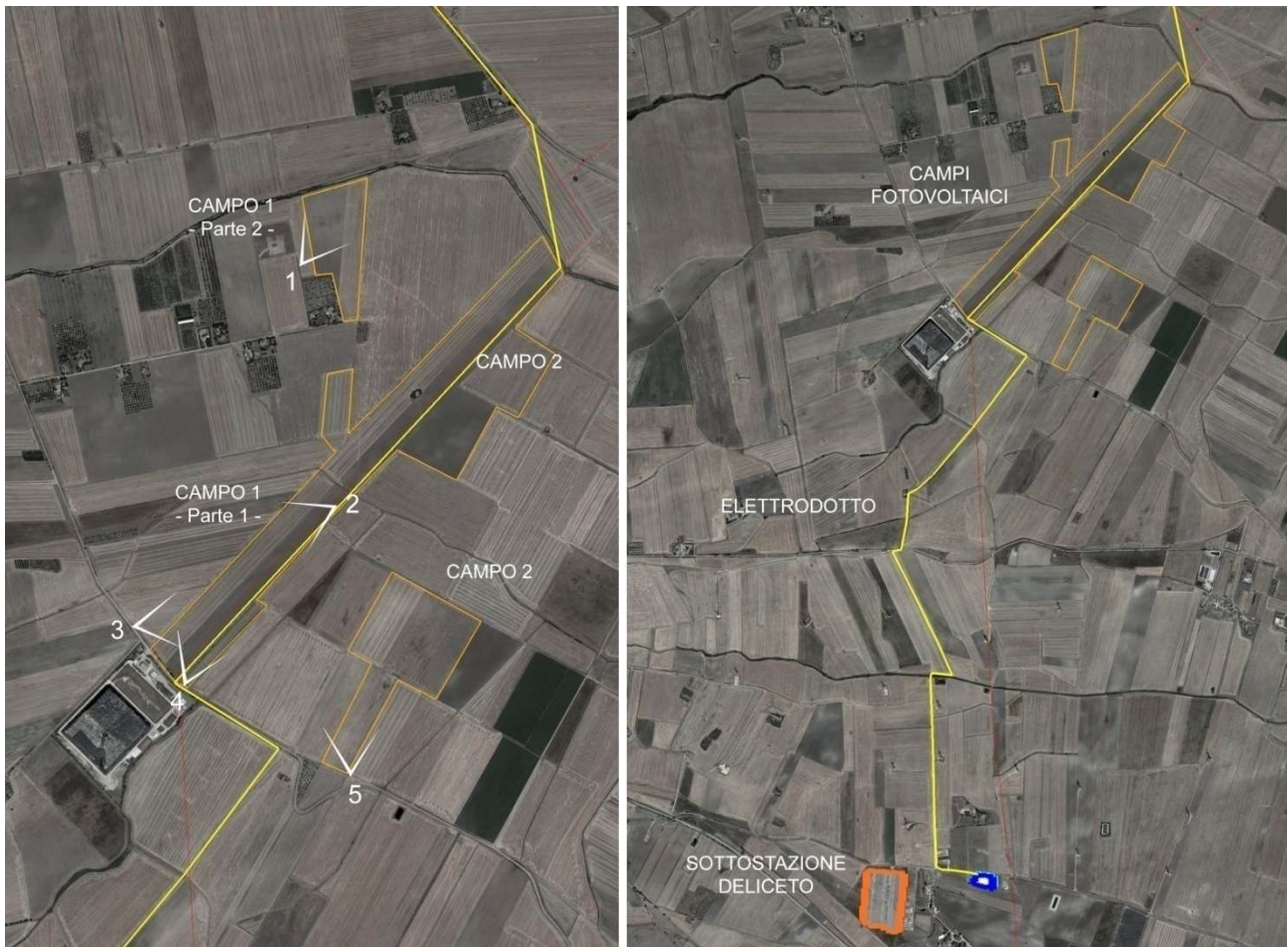
Figura 2: Vista aerea dell'area di impianto (Campo 1 e Campo 2), con coni visivi (a sx); vista del tracciato dell'elettrodotto interrato di collegamento alla sottostazione Terna S.p.A. (a dx).
