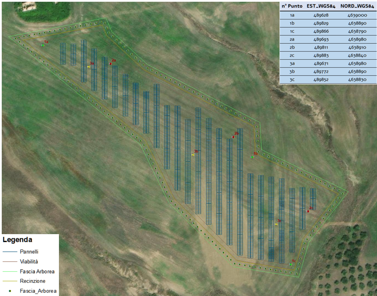
Figura 2.6. – Localizzazione e Coordinate WGS_1984_UTM_Zone_33N – EPSG 32633 dei punti di campionamento Area E.
