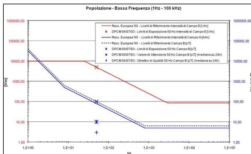
Figura 2.10. – Livelli esposizione Bassa Frequenza (1Hz – 100 kHz).
