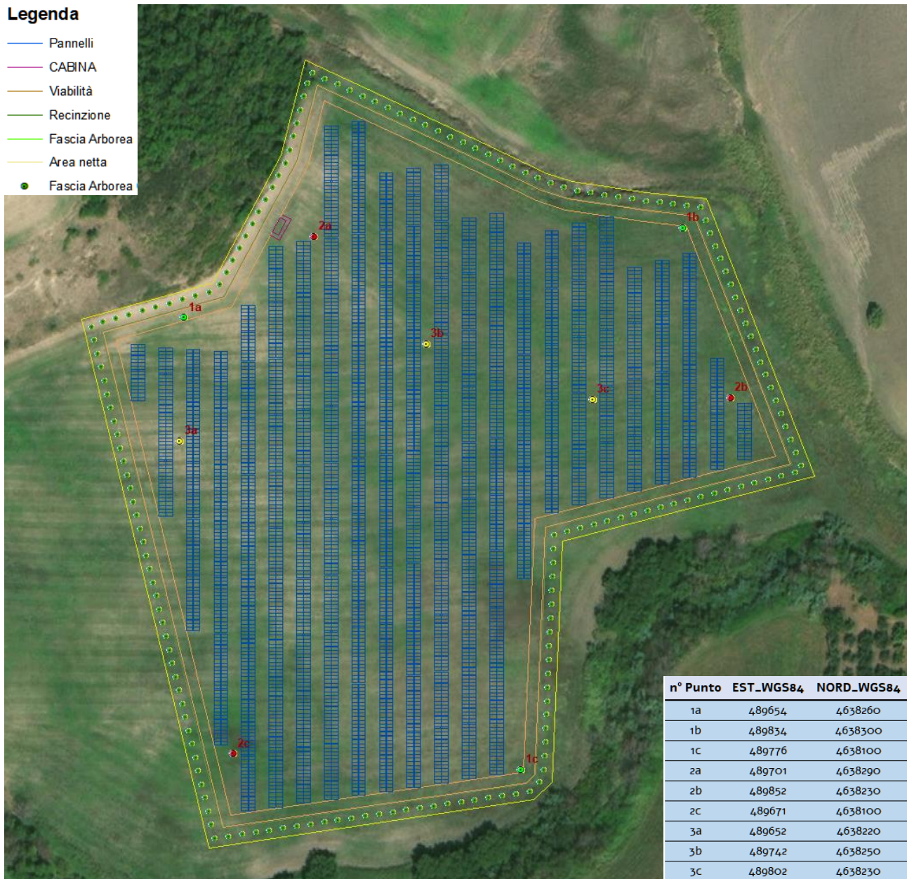
Figura 2.7. – Localizzazione e Coordinate WGS_1984_UTM_Zone_33N – EPSG 32633 dei punti di campionamento Area F.
