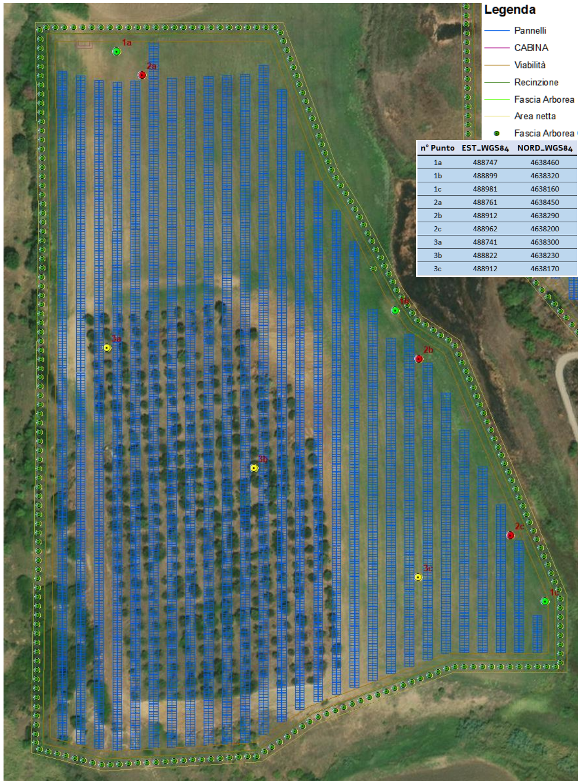
Figura 2.2. – Localizzazione e Coordinate WGS_1984_UTM_Zone_33N – EPSG 32633 dei punti di campionamento Area A.
