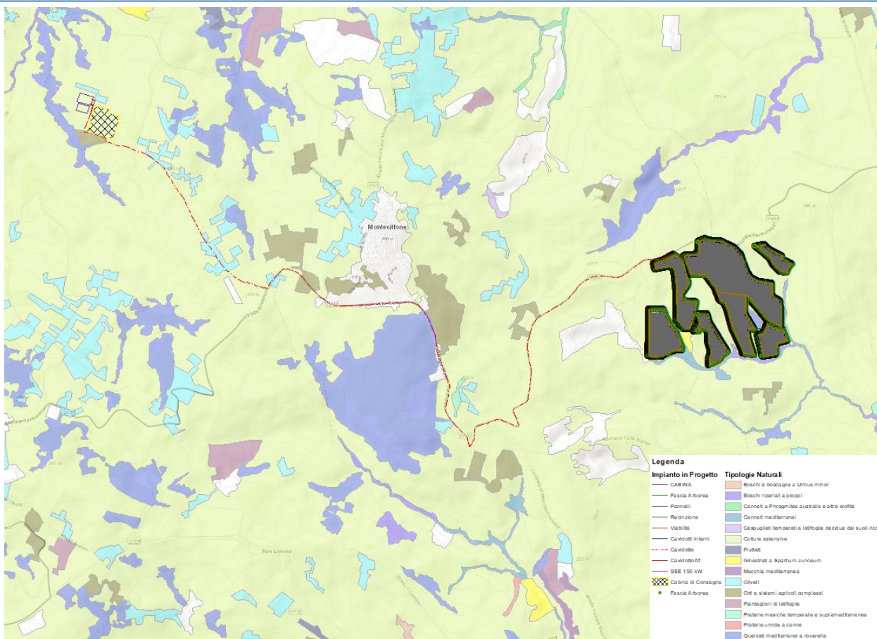
Figura 2.8. – Componenti naturali aree di progetto.
