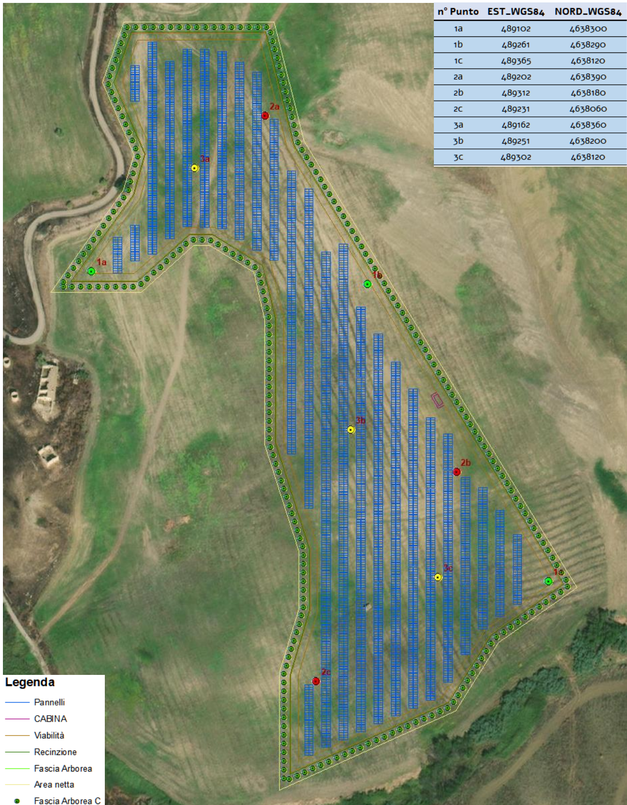
Figura 2.4. – Localizzazione e Coordinate WGS_1984_UTM_Zone_33N – EPSG 32633 dei punti di campionamento Area C.
