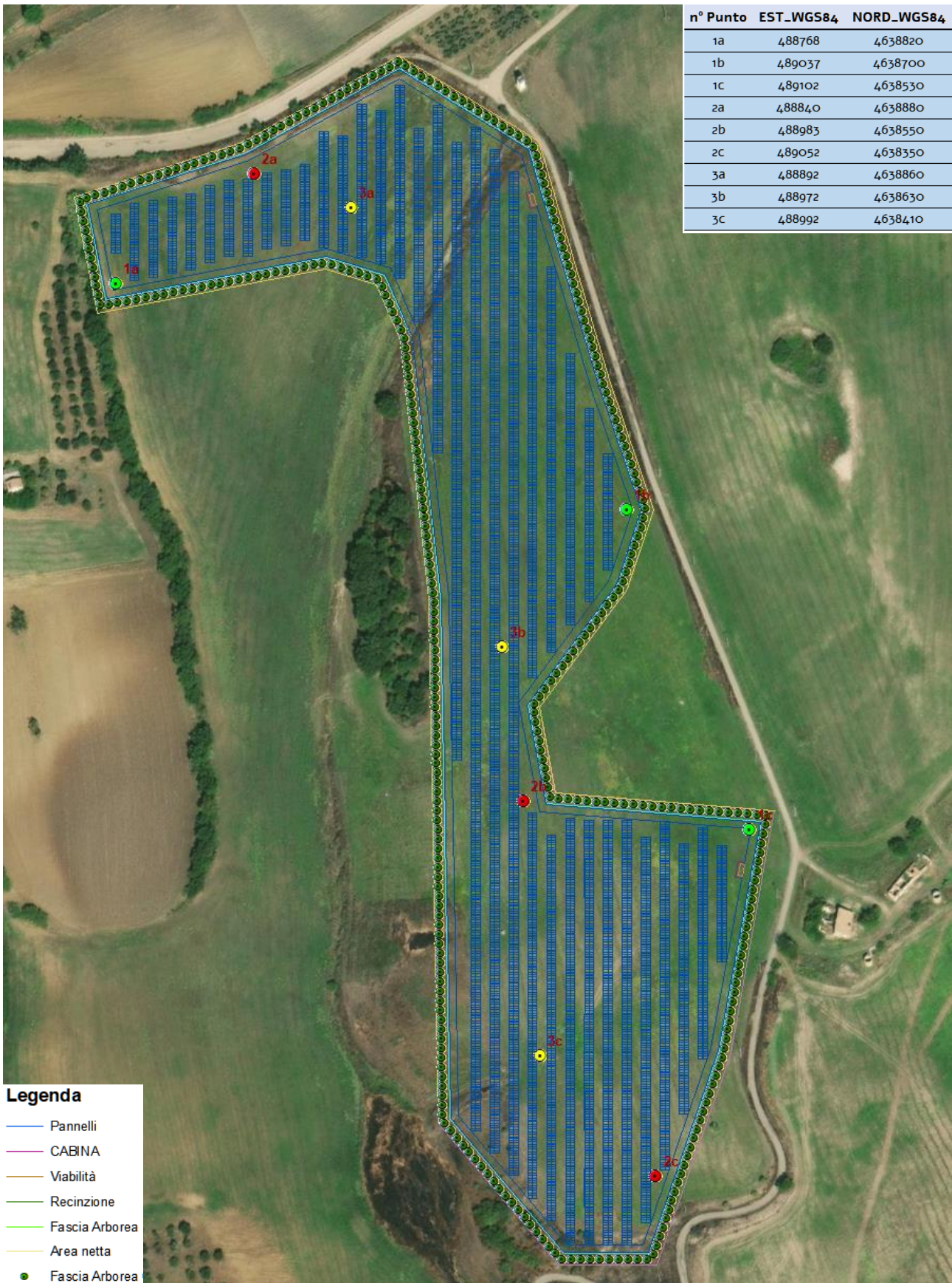
Figura 2.3. – Localizzazione e Coordinate WGS_1984_UTM_Zone_33N – EPSG 32633 dei punti di campionamento Area B.
