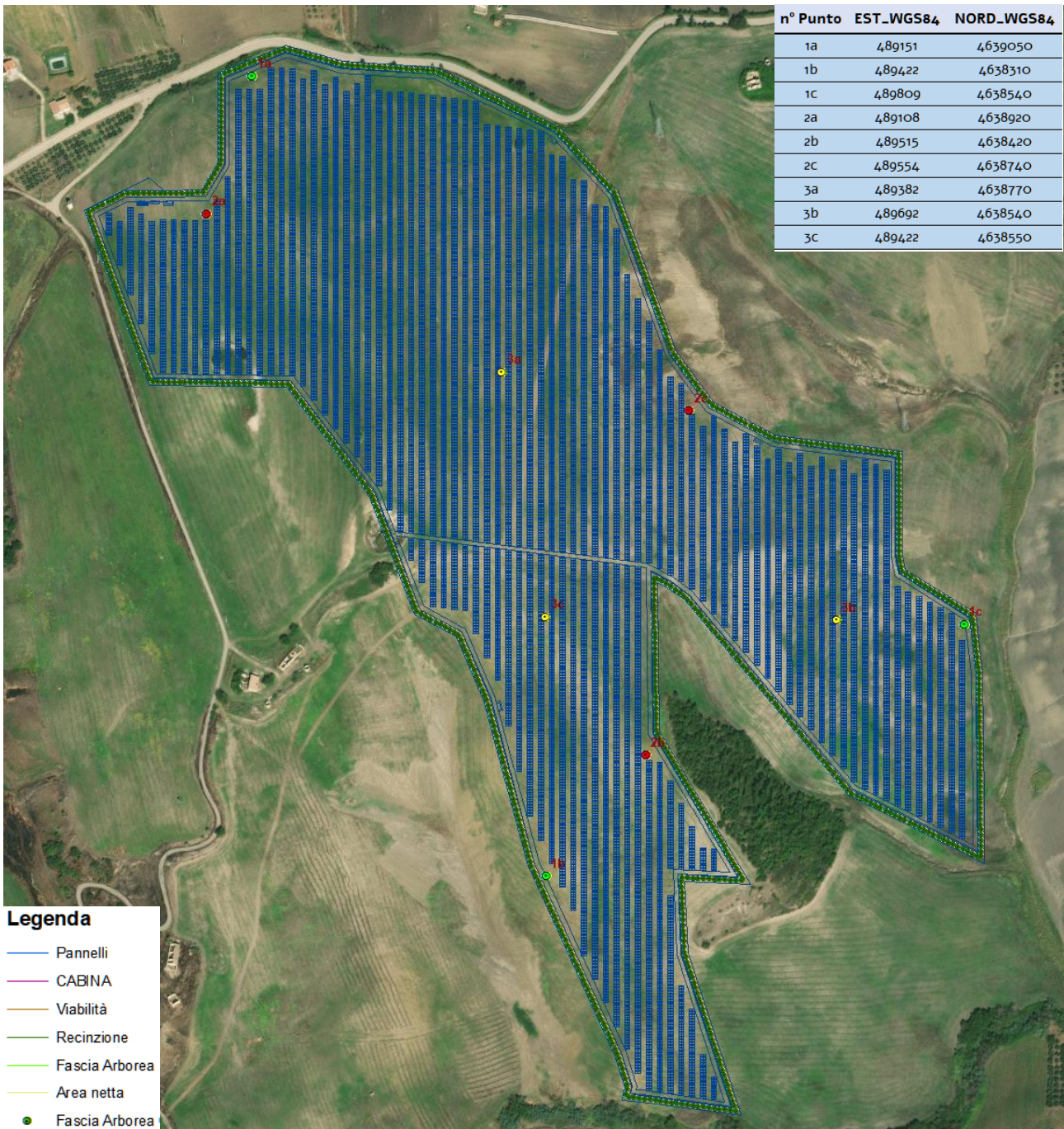
Figura 2.5. – Localizzazione e Coordinate WGS_1984_UTM_Zone_33N – EPSG 32633 dei punti di campionamento Area D.
