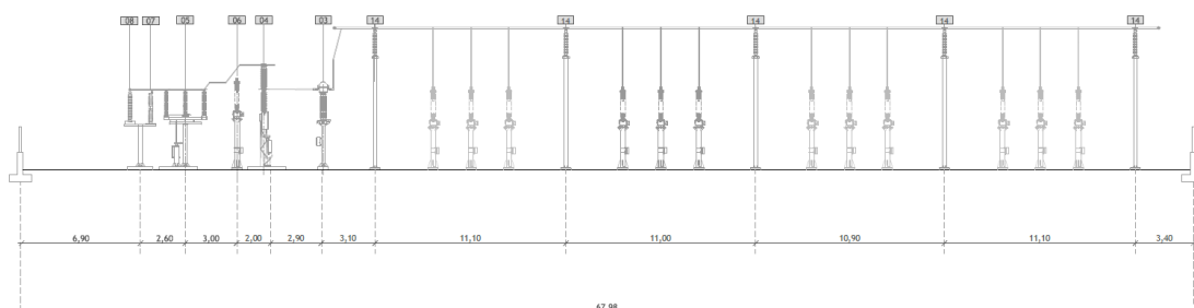
Figura 12. Sezione elettromeccanica
