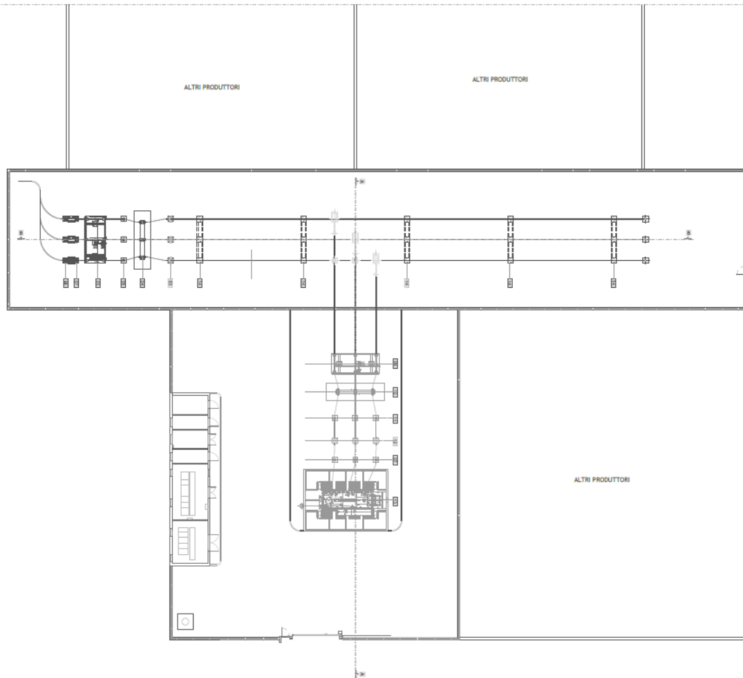
Figura 11. Planimetria elettromeccanica
