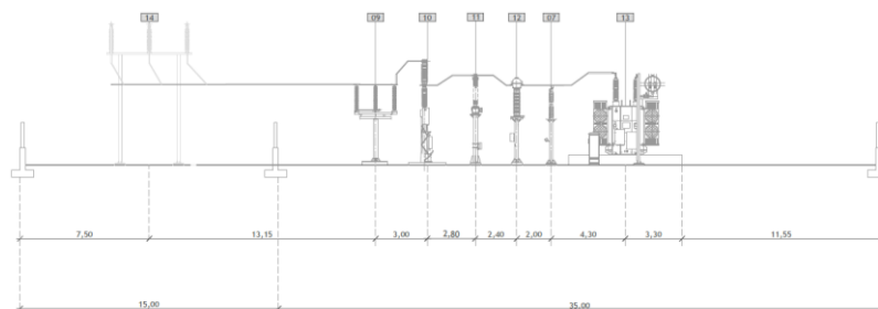
Figura 12. Sezione elettromeccanica
