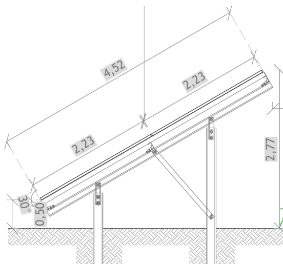
Figura 4. Particolare costruttivo
