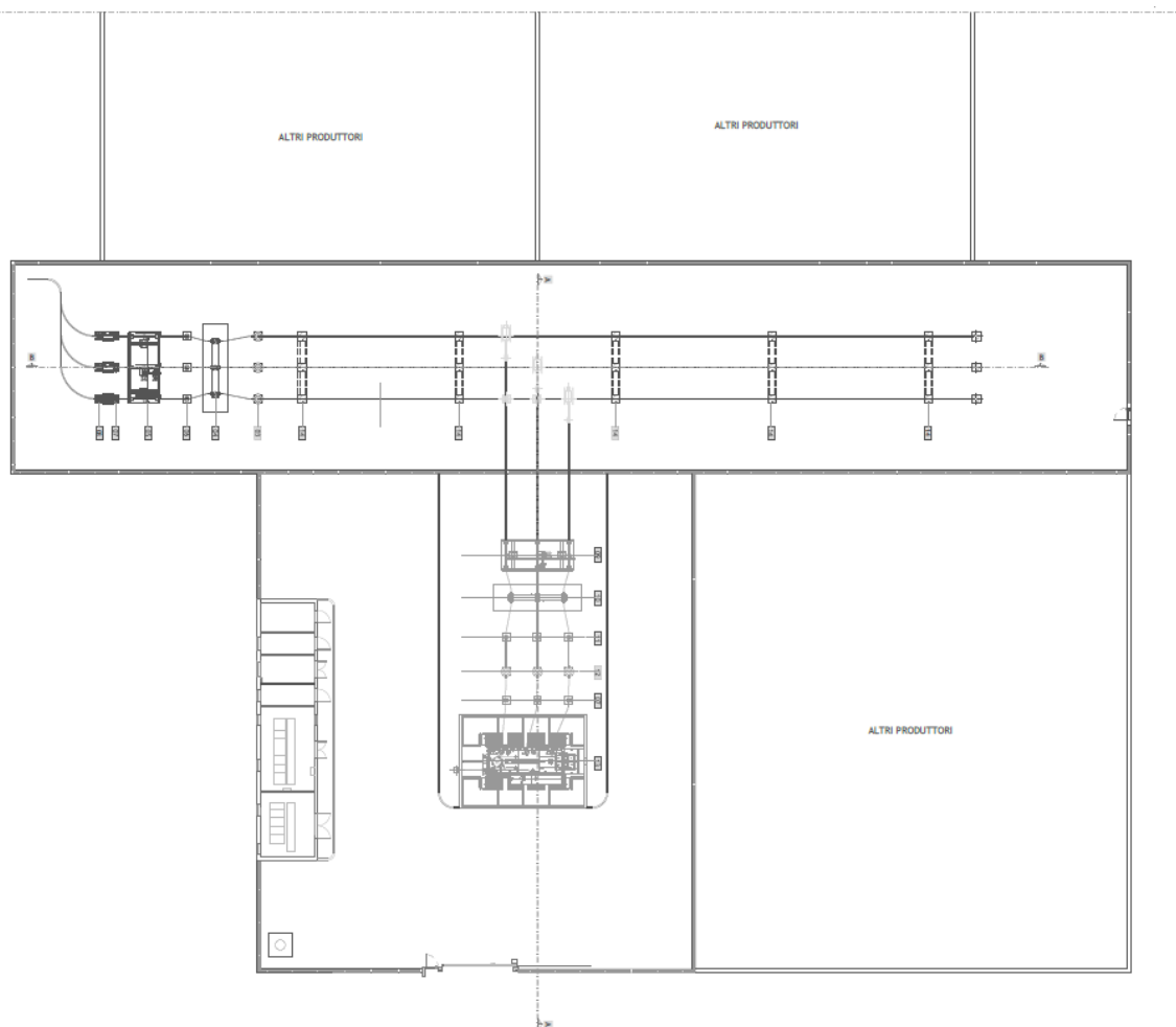
Planimetria Elettromeccanica
