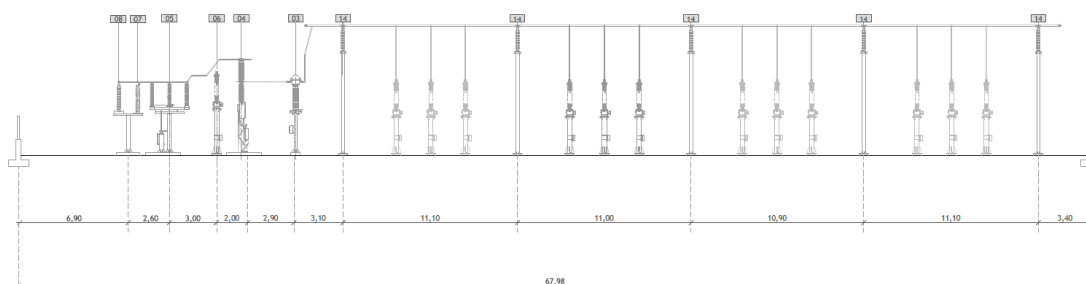
Sezioni Elettromeccaniche
