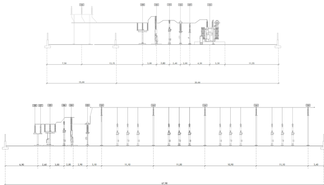
Sezioni Elettromeccaniche
