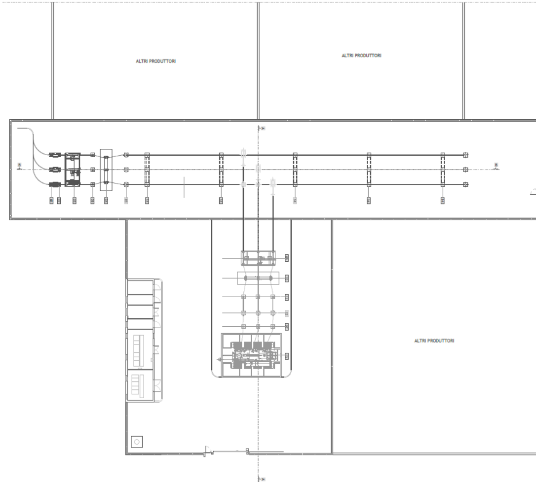
Planimetria Elettromeccanica
