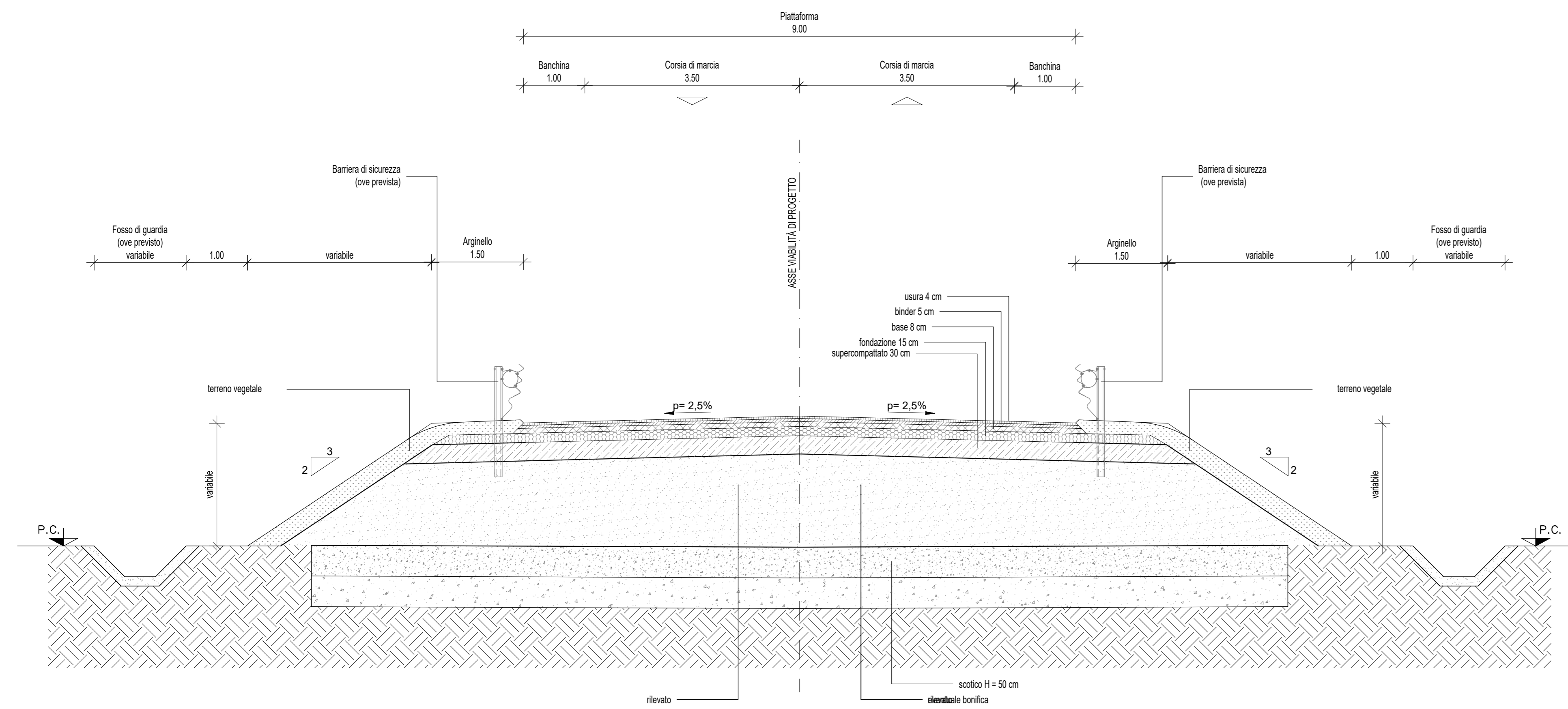
SEZIONE TIPO STRADALE NV04 CATEGORIA F LOCALI - "F1" EXTRA-URBANA IN RETTIFILIO - IN RILEVATO SCALA 1:50
