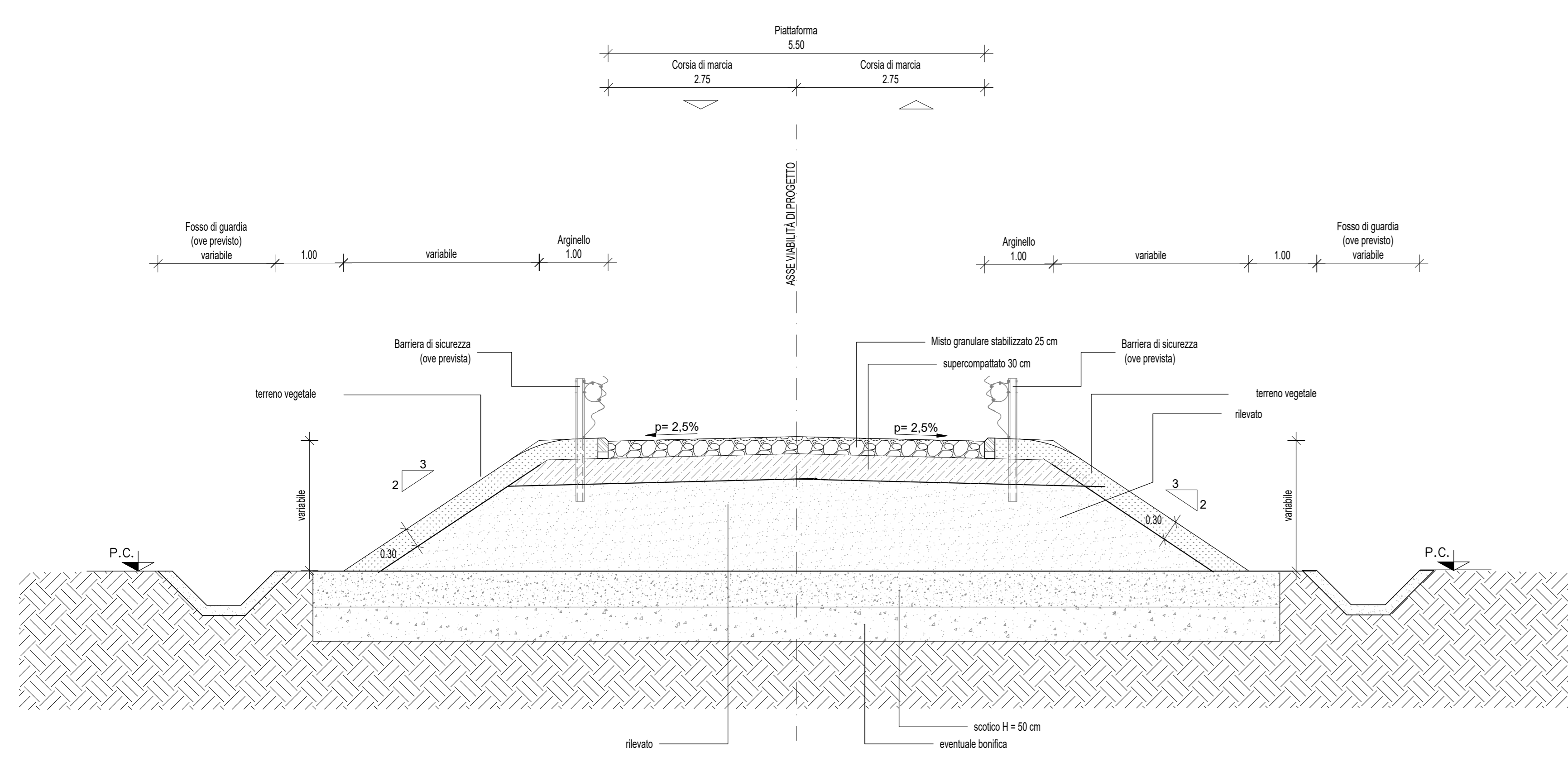
SEZIONE TIPO STRADALE NV09 CATEGORIA F LOCALI - VIABILITÀ A DESTINAZIONE PARTICOLARE L=5.50m IN RETTIFILLO - IN RILEVATO SCALA 1:50
