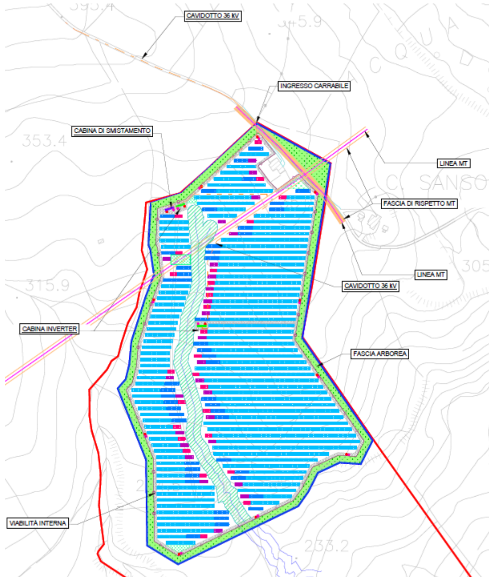
Figura 11 - Layout di impianto Sottocampo 1
