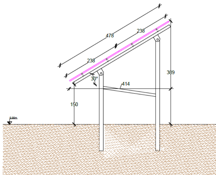
Figura 15 - Particolare strutture di fissaggio
