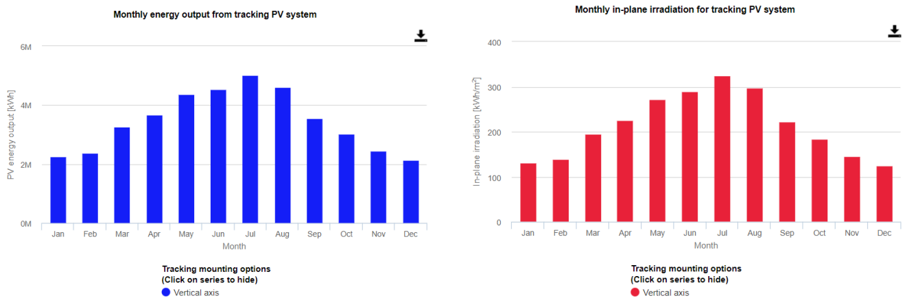
Figura 7 – Energia e Irraggiamento mensile nel piano di inseguimento
