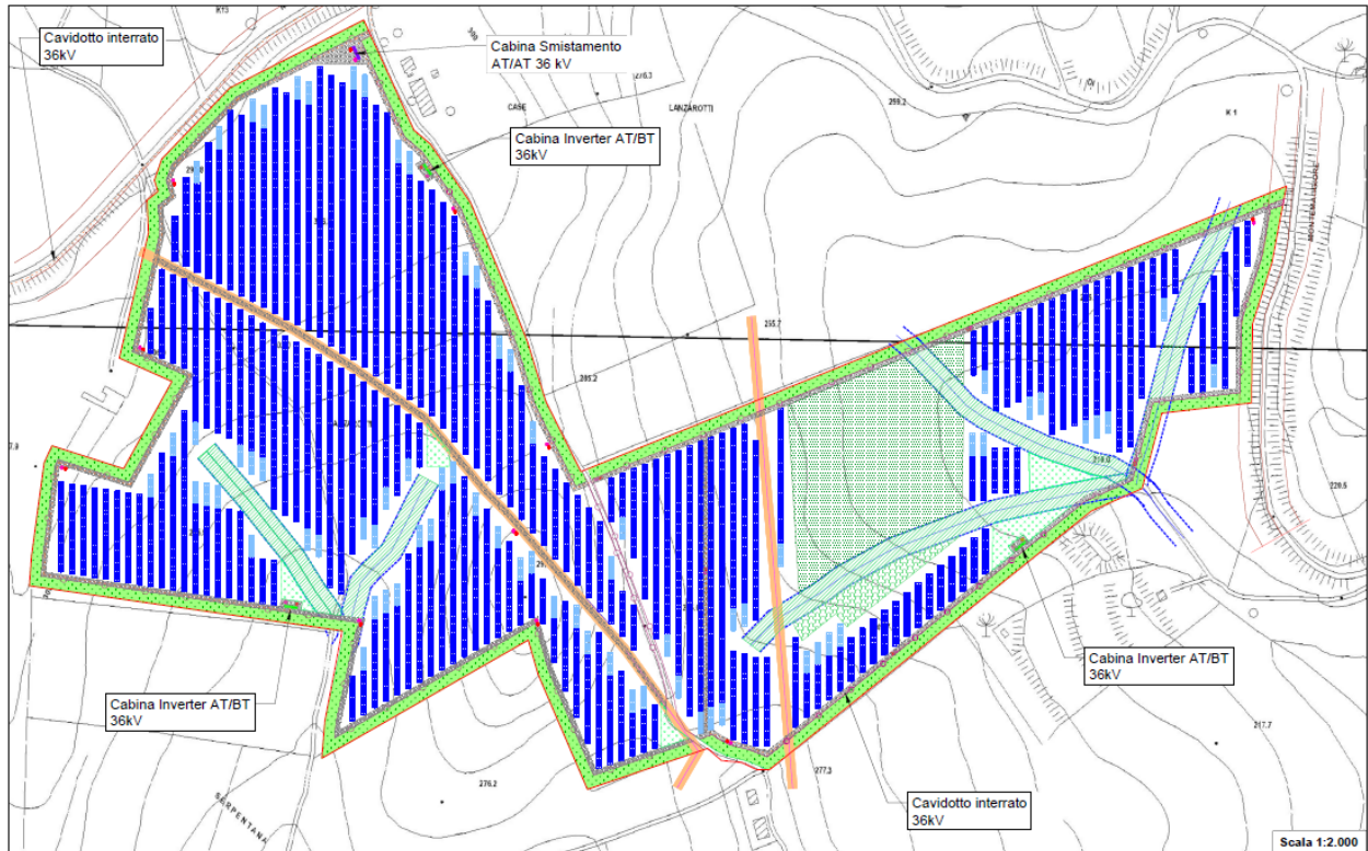
Figura 12 - Layout di impianto Sottocampo 2-3
