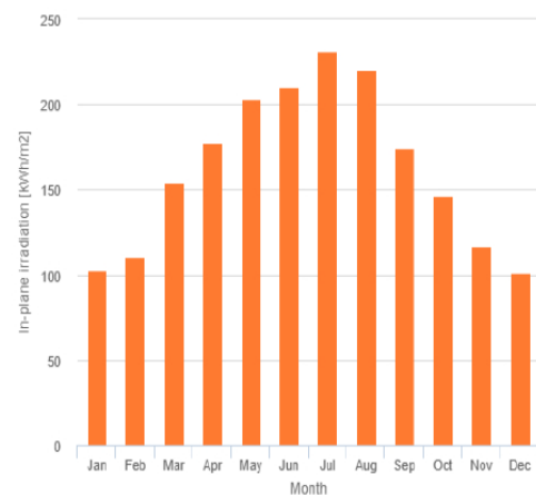
Figura 6 – Energia ed Irraggiamento mensile sul piano fisso [kWh/m²]
