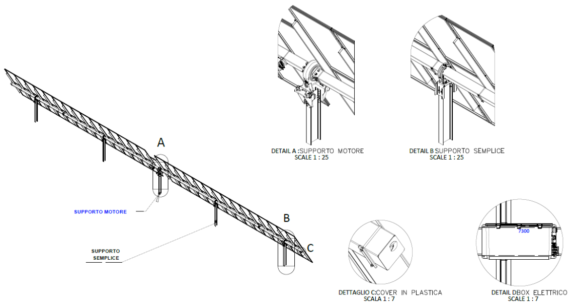
Figura 16 - Particolari Tracker
