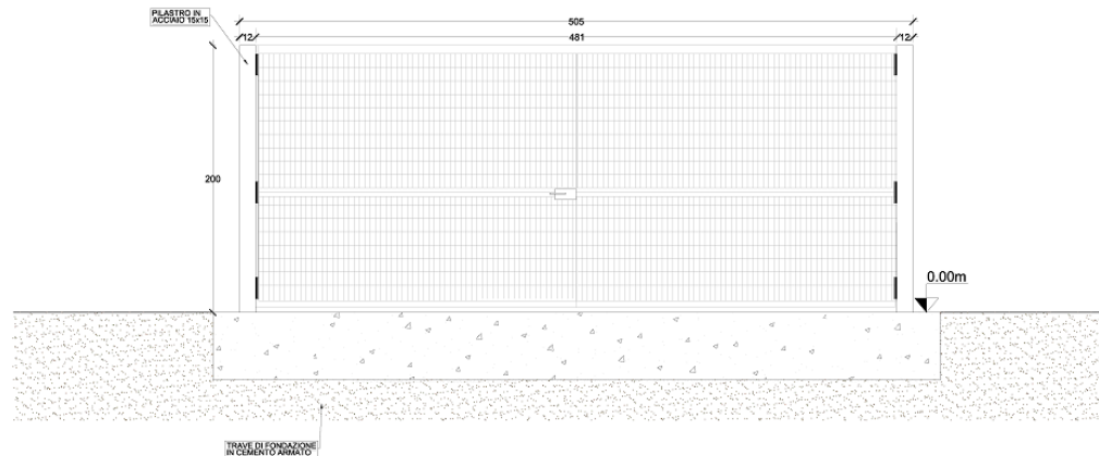
Figura 14 - Particolare cancello di ingresso
