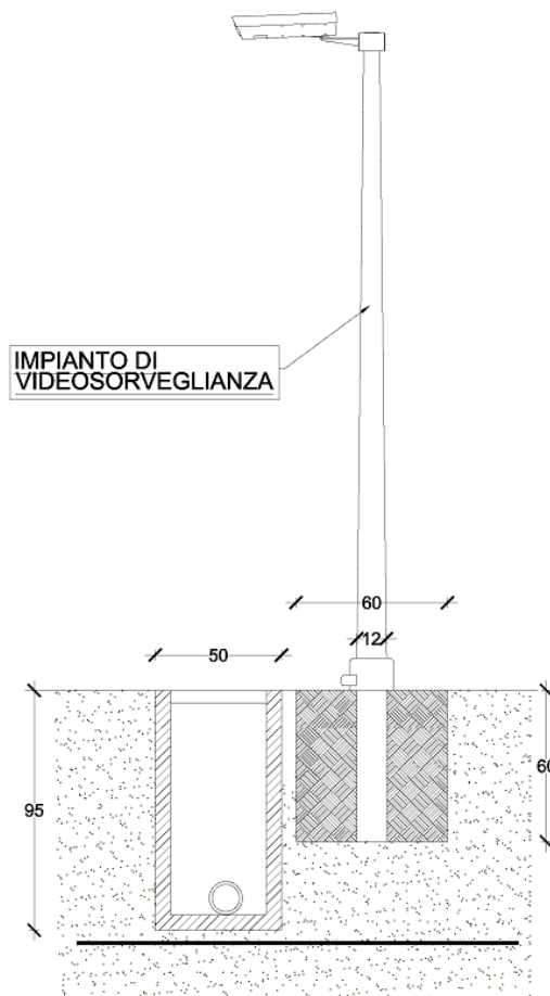
Figura 17 - Palo per l'impianto di videosorveglianza
