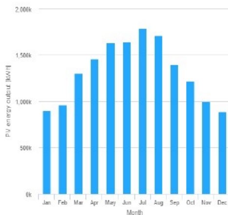
Figura 10 - Energia e Irraggiamento mensile nel piano fisso
