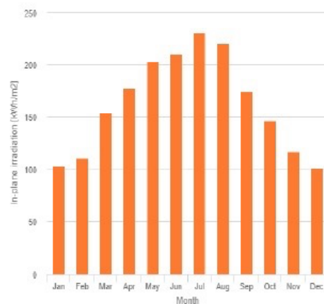
Figura 10 - Energia e Irraggiamento mensile nel piano fisso
