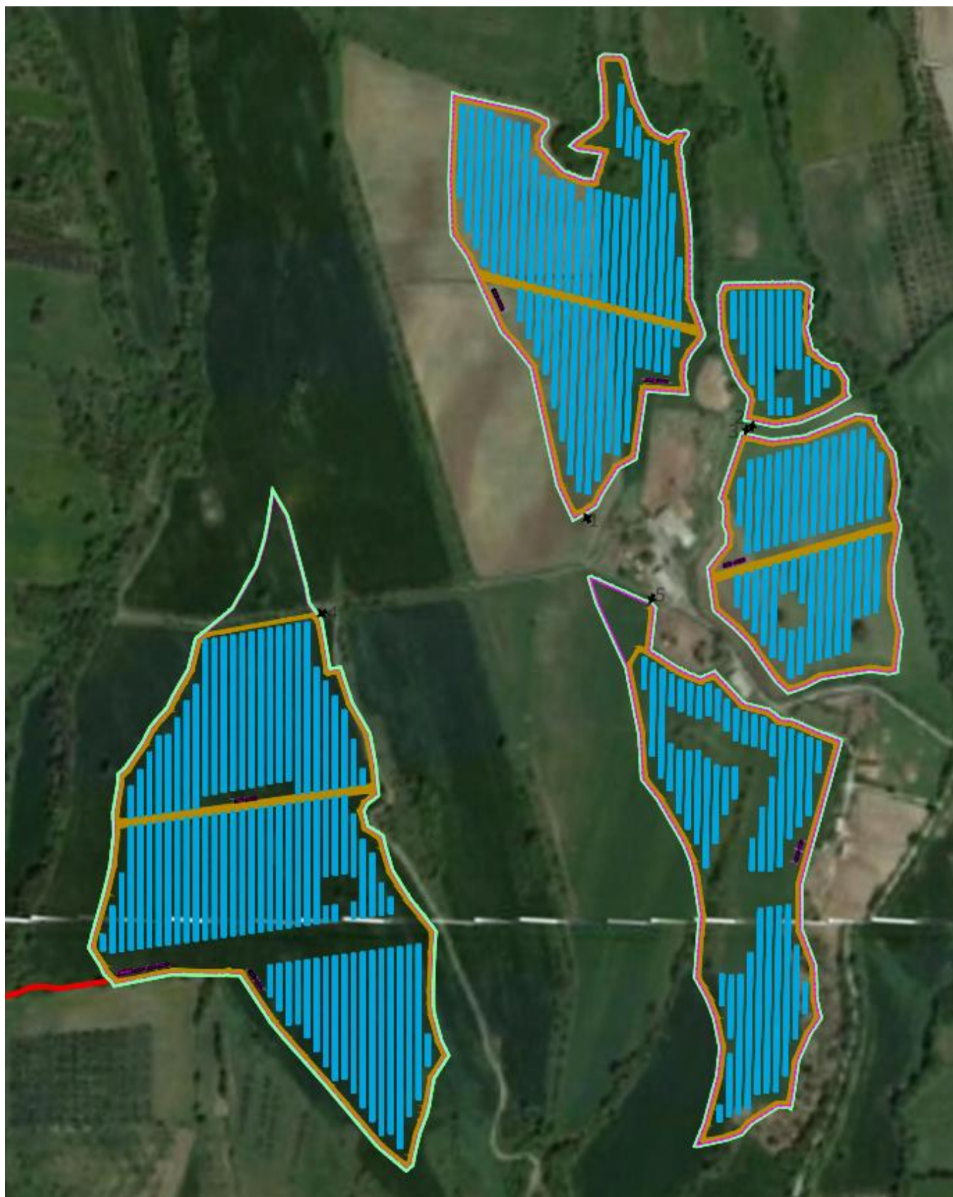
Figura 2 - inquadramento ortofoto
