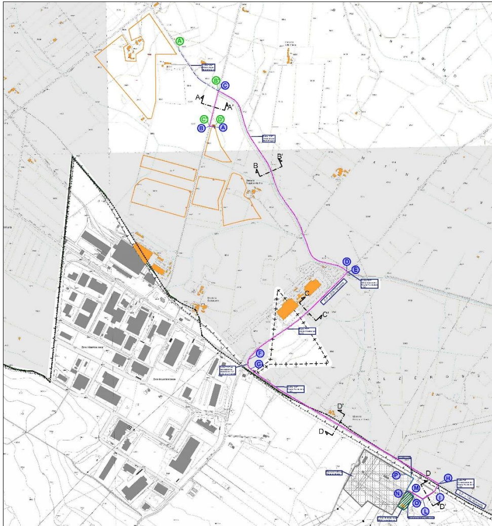
Percorso cavidotto MT di connessione suddiviso in tratte
