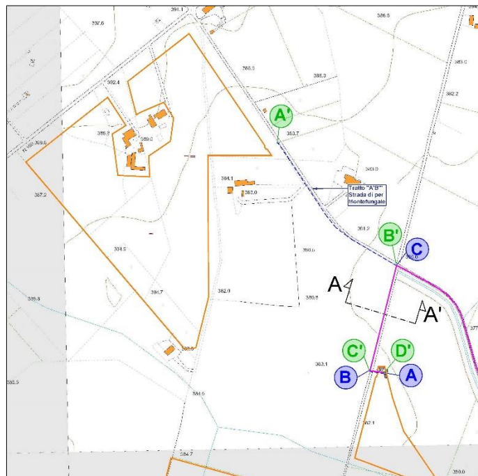
Cavidotto di connessione tra il Lotto 1 e la cabina di raccolta
