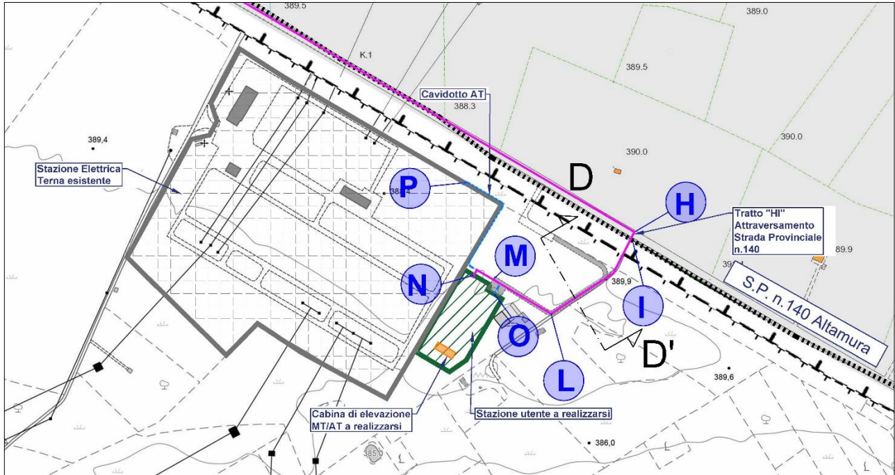
Percorso cavidotto AT di connessione alla SE "MATERA"
