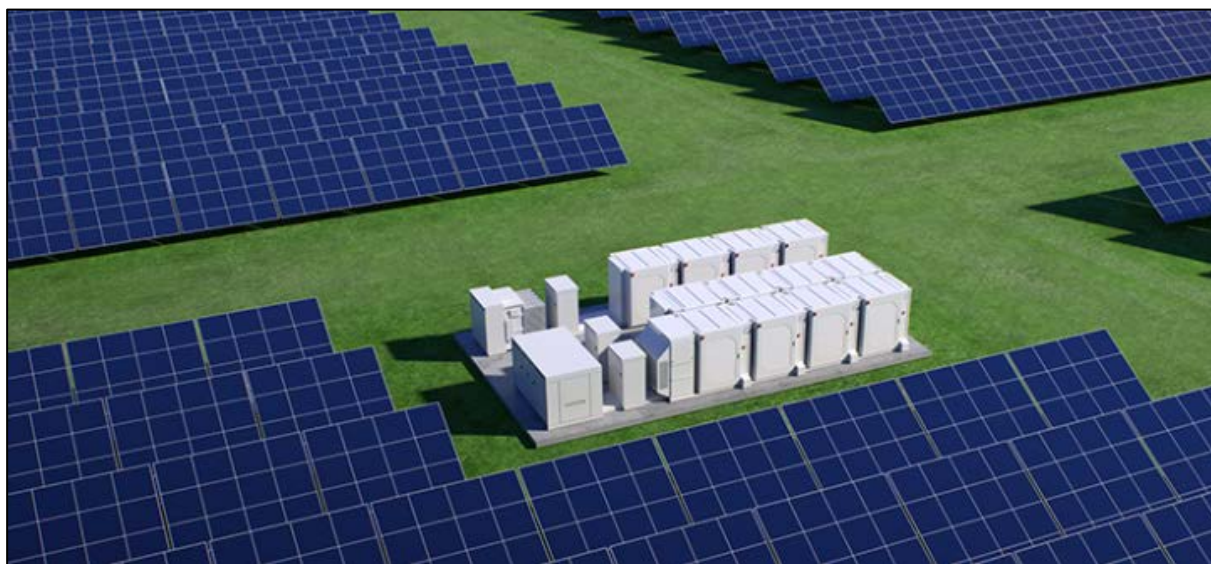
Figura 35: esempio di sistema di stoccaggio per impianto fotovoltaico - Sunstack
