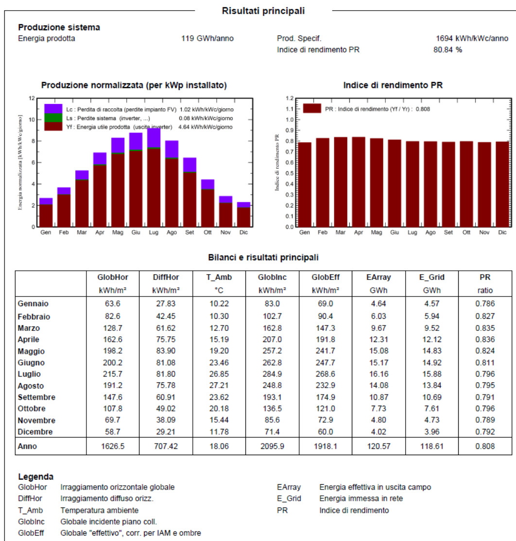
Figura 3: risultati ottenuti con PVSyst
