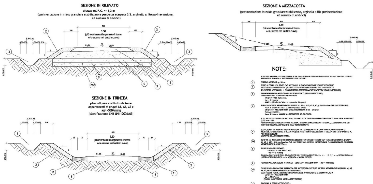
Figura 32: dettagli relativi alle caratteristiche costruttive della viabilità interna al parco
