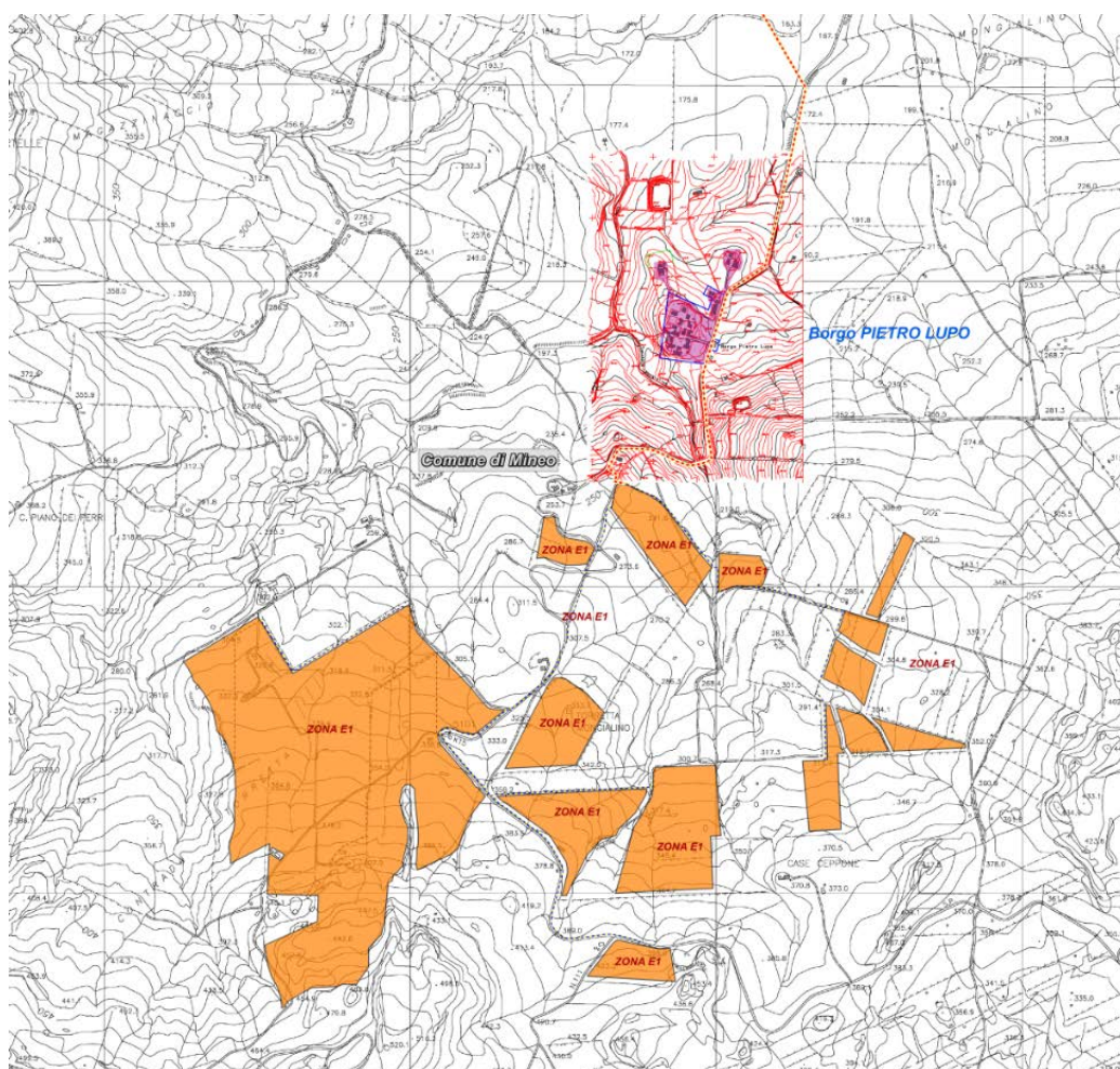
Figura 24: PRG con individuazione del parco agrovoltaico di Mineo (CT) in località “Contrada Torretta” e “Torretta Mongialino” – stralcio dell’elaborato grafico “Inquadramento urbanistico”
