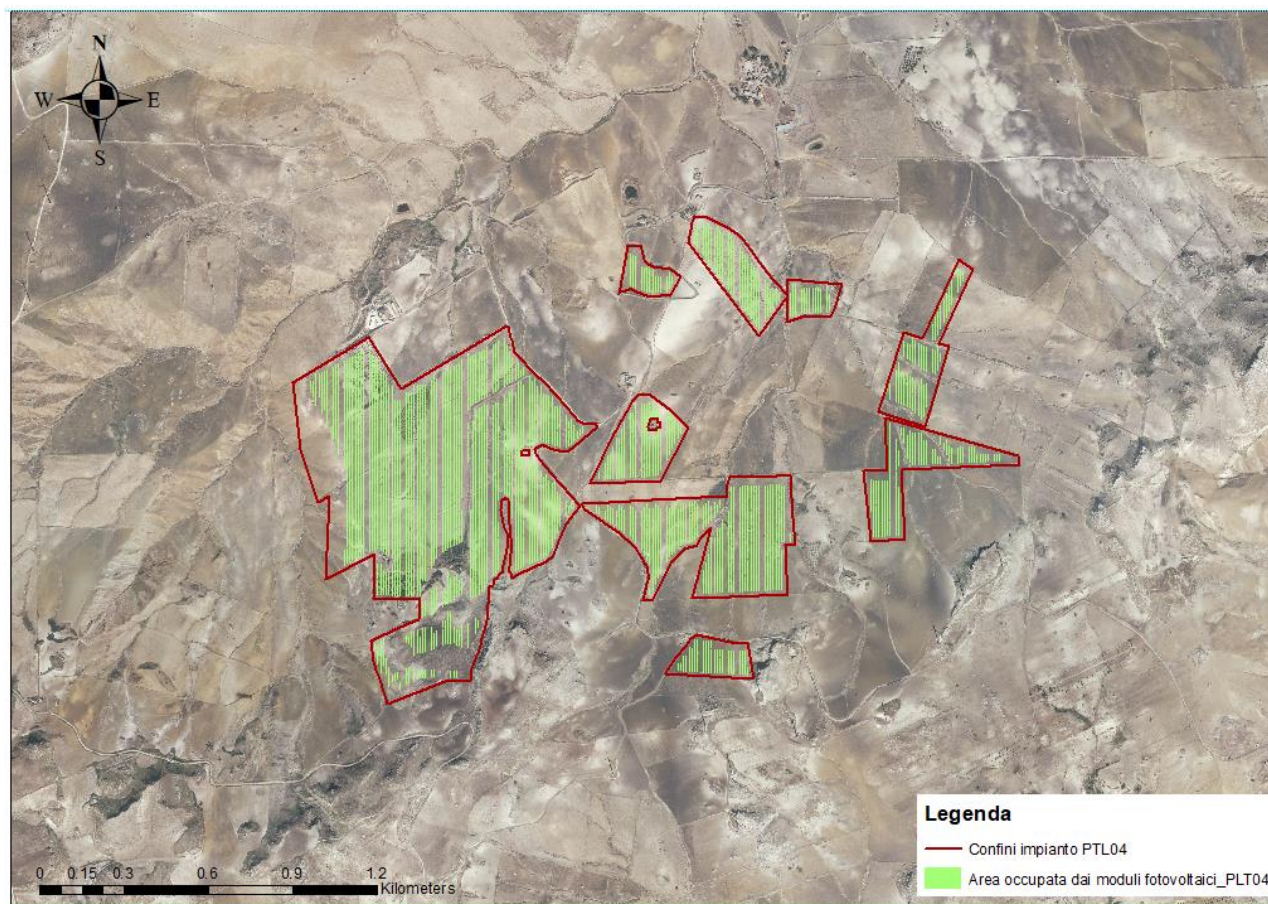
Figura 4: Layout di progetto
