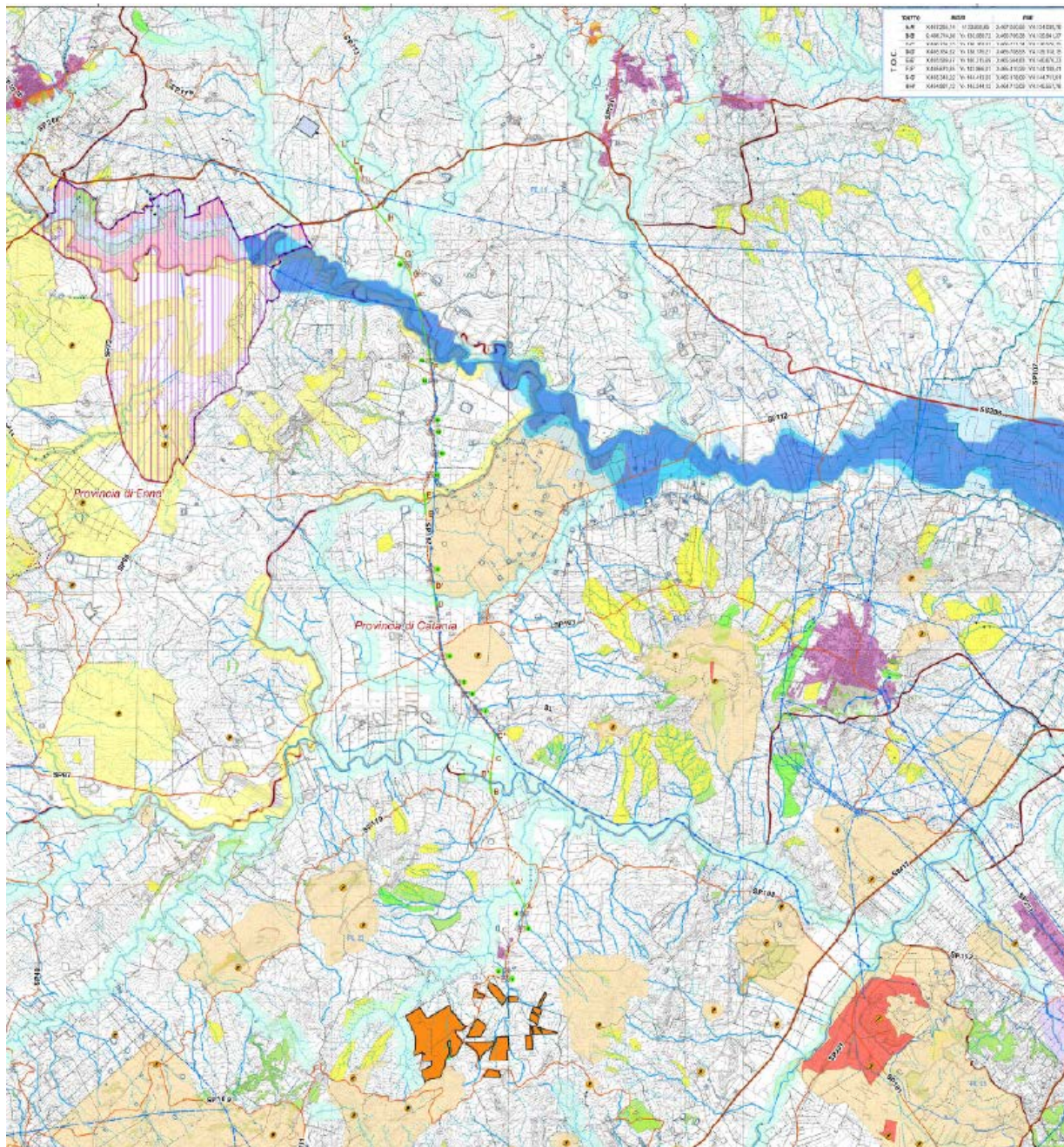
Figura 31: interferenze del parco di Mineo (CT), da realizzare in località "Contrada Torretta" e "Torretta Mongialino", con le infrastrutture presenti.
