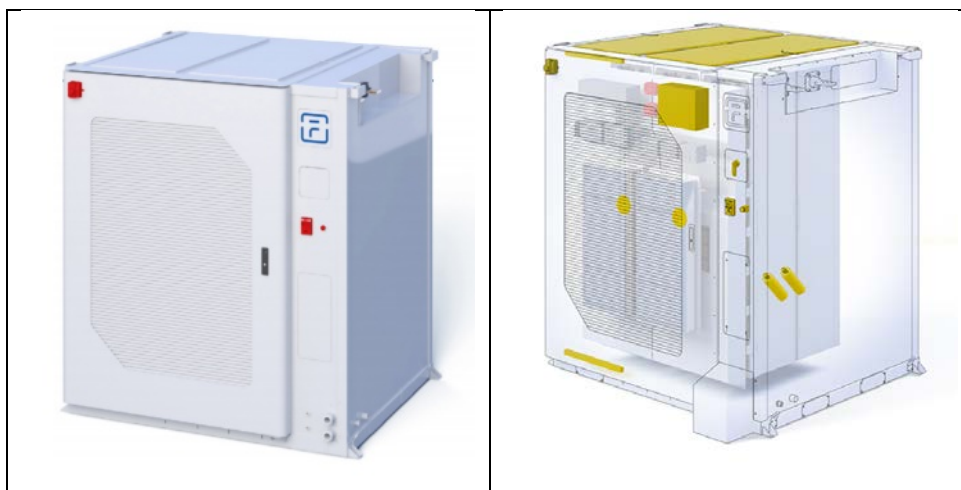
Figura 4: componente modulabile del sistema di Storage: il Cube
