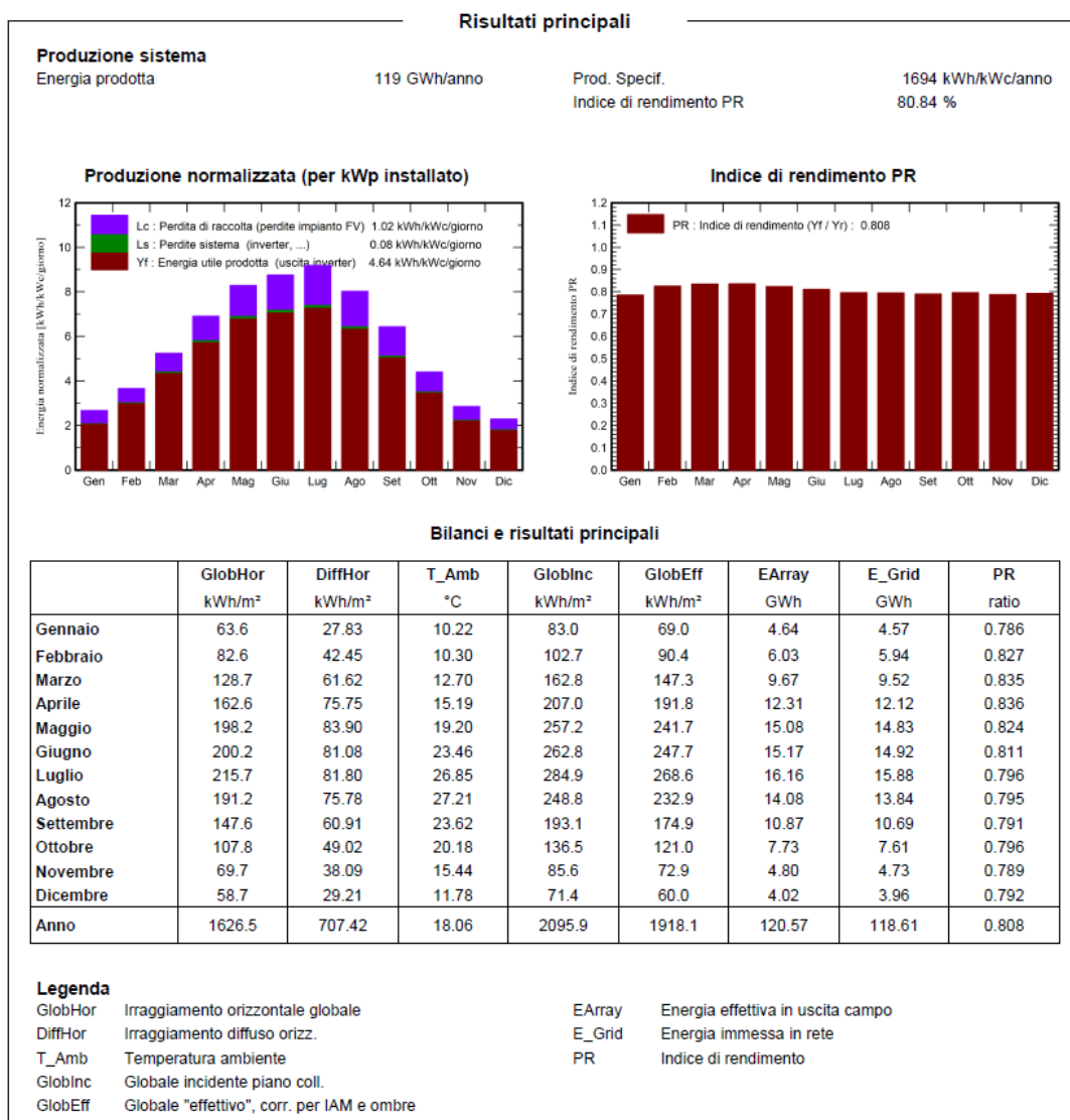
Figura 10: risultati ottenuti con PVSyst
