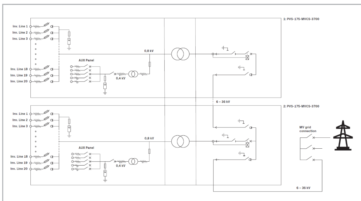
Figura 5: Esempio di diagramma della "PVS-175-MVCS"
