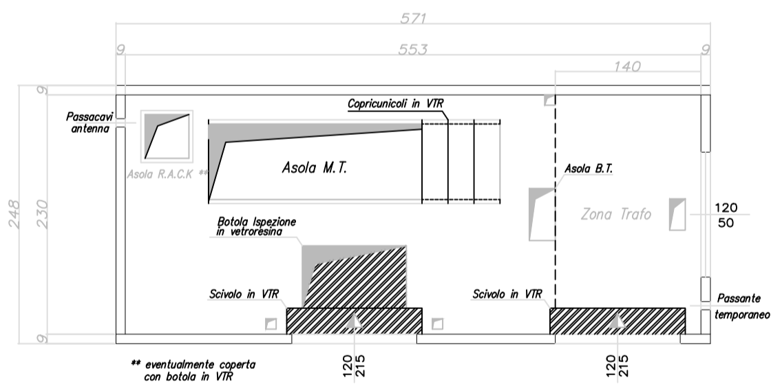
PIANTA
