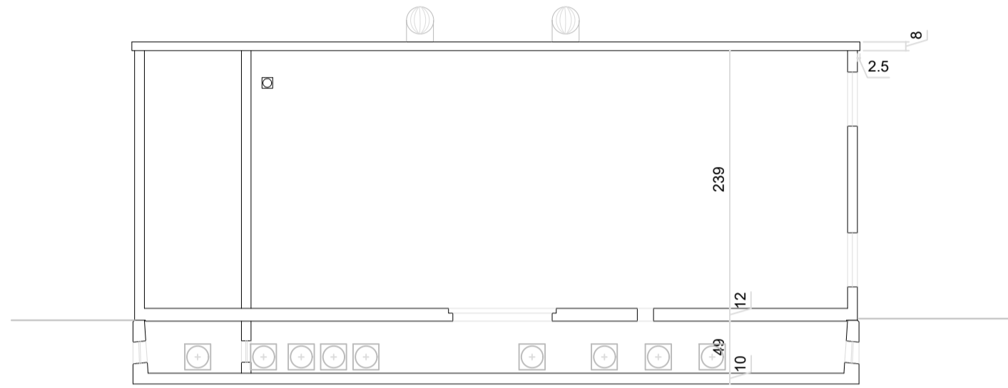
sezione X-X
