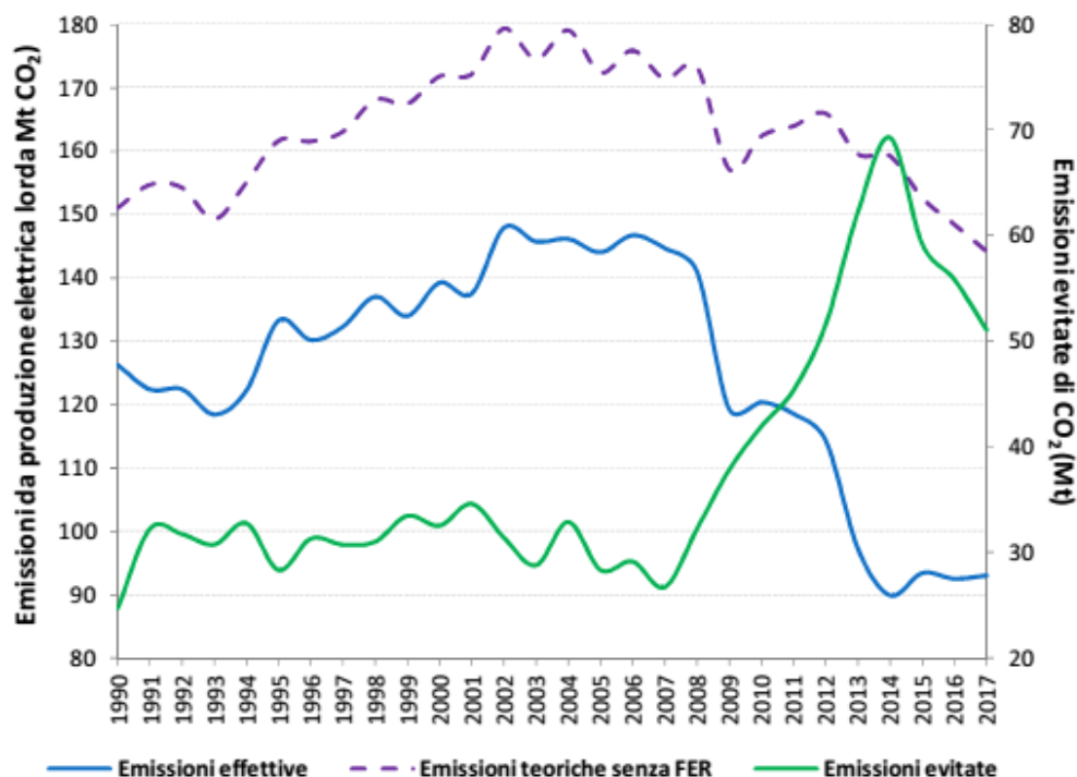
Figura 9 Andamento delle emissioni effettive per la produzione lorda di energia elettrica e delle emissioni teoriche per la produzione di energia elettrica da fonti rinnovabili con equivalente produzione da fonti fossili.
