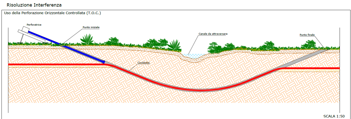
Figura 22 Rappresentazione schematica della Trivellazione Orizzontale Controllata (T.O.C.). I punti di infissione saranno esterni alla fascia di rispetto fluviale identificati dallo studio.
