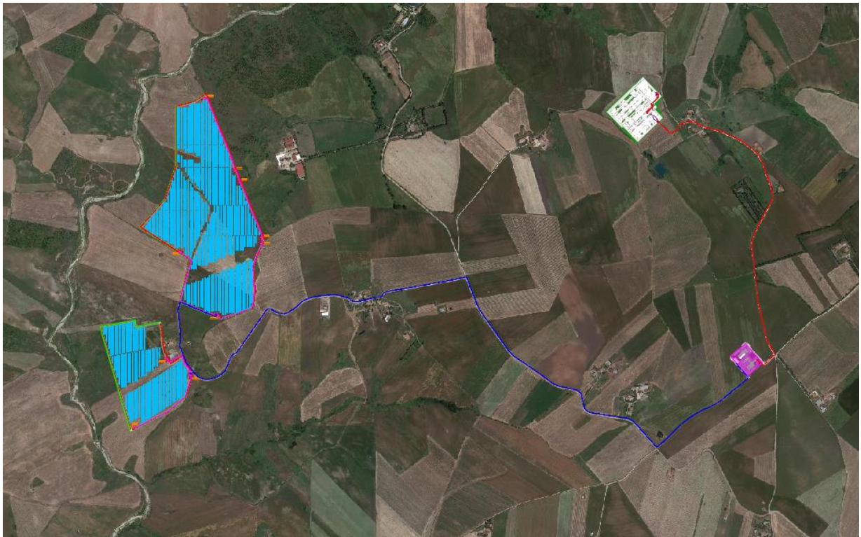
Figura 2 Stralcio elaborato DEF-TAV.04 – Layout su ortofoto
