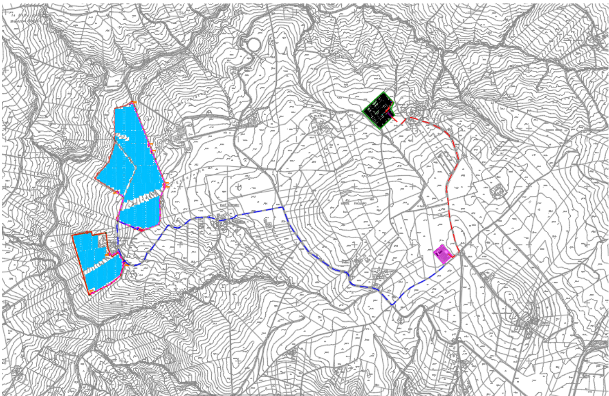
Figura 3 Stralcio elaborato DEF-TAV.05 – Layout su CTR
