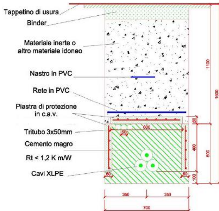
Figura 18 Sezione tipo di posa dei cavi elettrici
