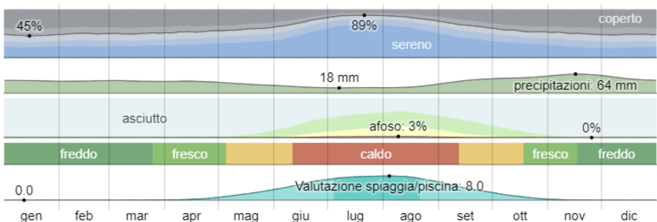
Figura 5 Sommario climatico
