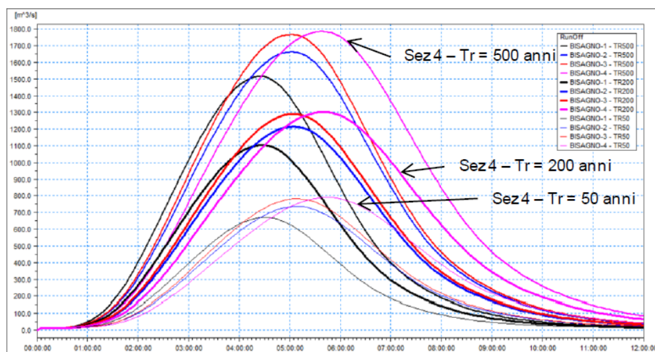
Figure 3 Igrammi di assegnato tempo di ritorno TR relativi al torrente Bisagno calcolati con il modello idrologico (estratto da DHI-ART).
