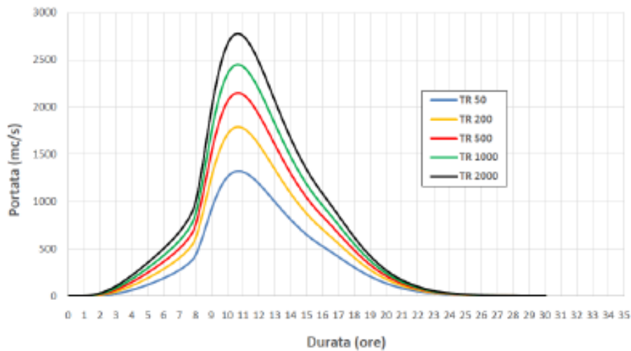
Figure 2 Torrente Polcevera: idrogrammi di piena per assegnati tempi di ritorno (estratto da ITALFERR-RINA)
