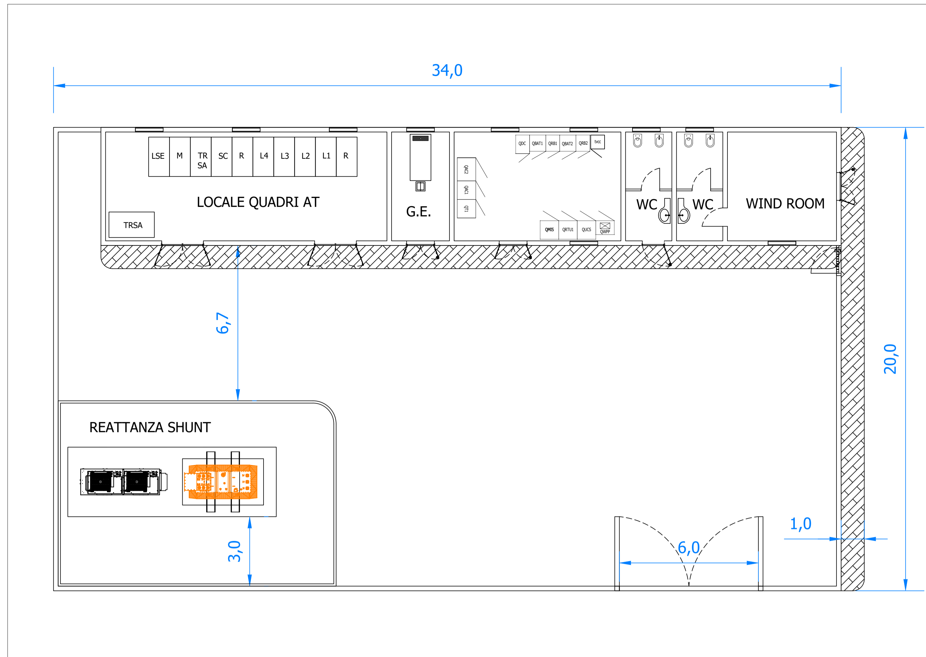
Planimetria cabina utente - Scala 1:100
