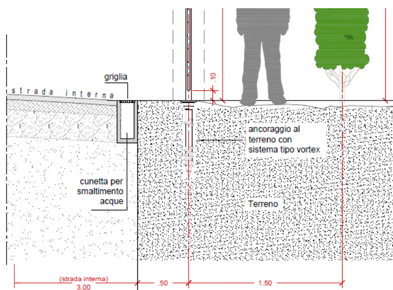
Schema impianto smaltimento acque meteoriche perimetrale
