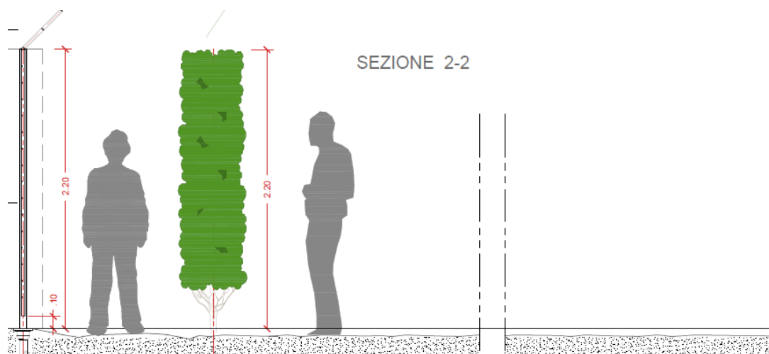
Prospetto recinzione perimetrale con mitigazione – sistema adottato
