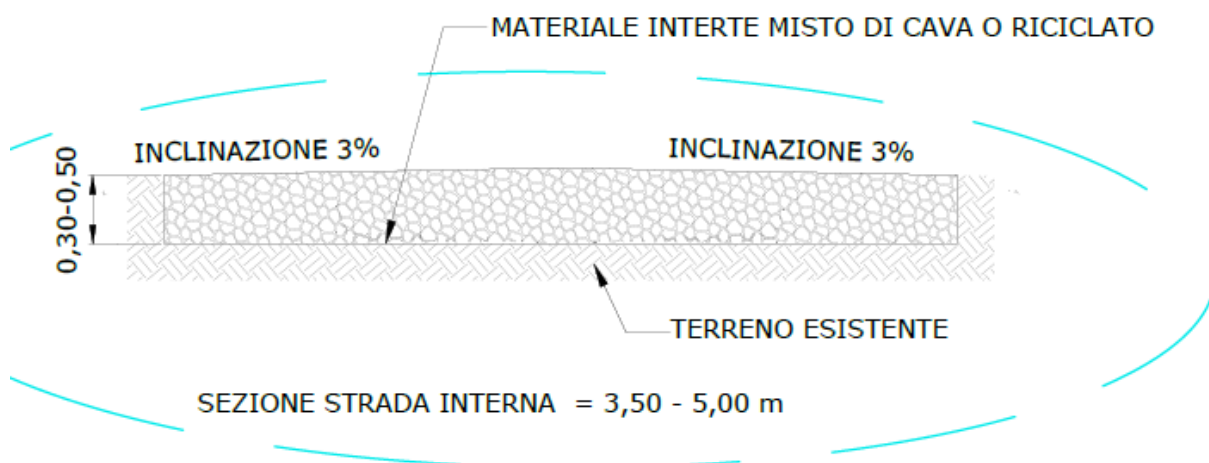
Fig. 17 – Viabilità interna
