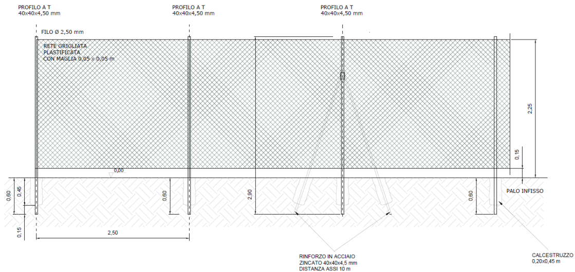
Fig. 15 – Recinzione perimetrale
