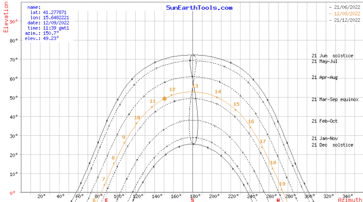
Fig. 26 - Diagramma Solare Polare (Orta Nova)
