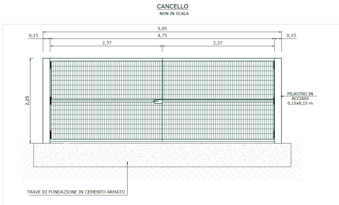
Fig. 16 – Cannello a doppia anta
