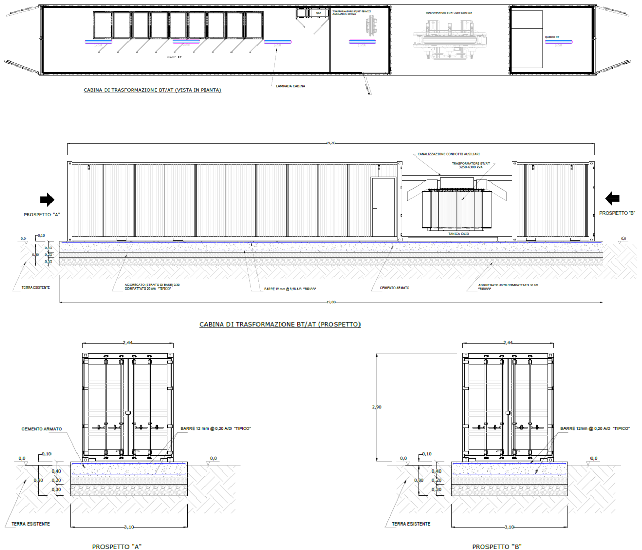
Fig. 19 - Cabina di trasformazione BT/AT
