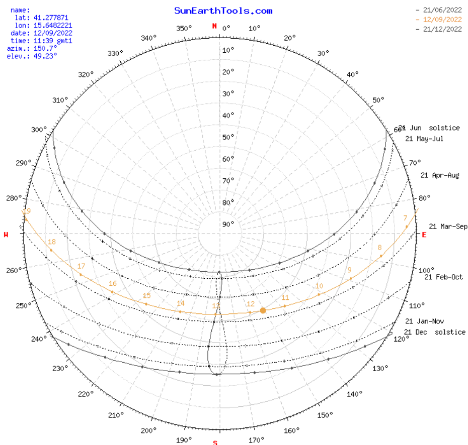
Fig. 25 - Diagramma Solare Polare (Orta Nova)
