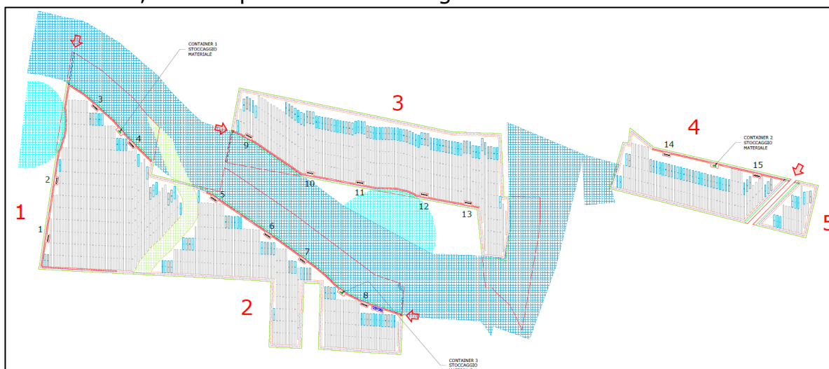
Fig. 7 - Layout di impianto
