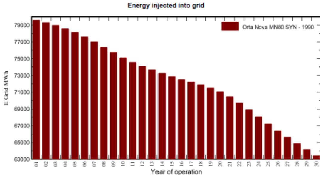
Fig. 28 – Producibilità dell’impianto con degrado moduli (30 anni)
