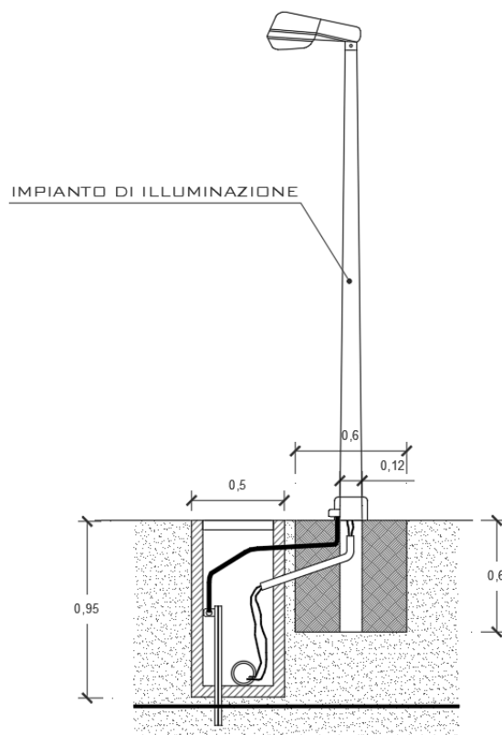
Fig. 23 – Sistema di illuminazione
