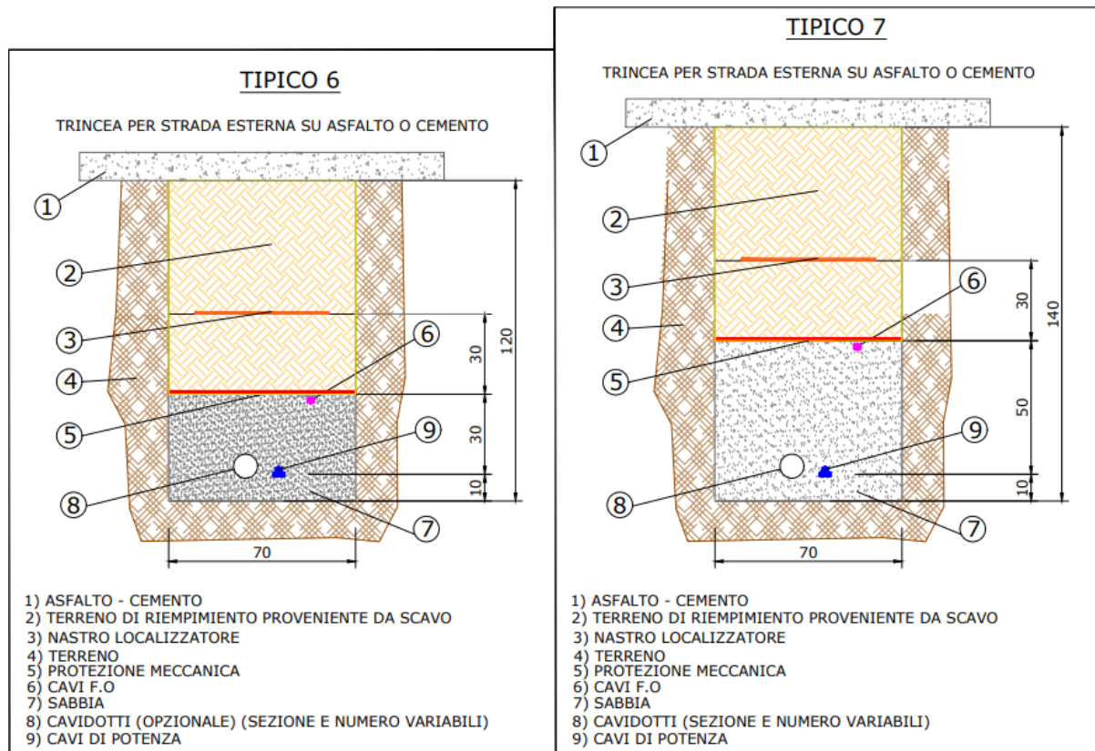
Fig. 18 – Tipici scavi e posa cavi
