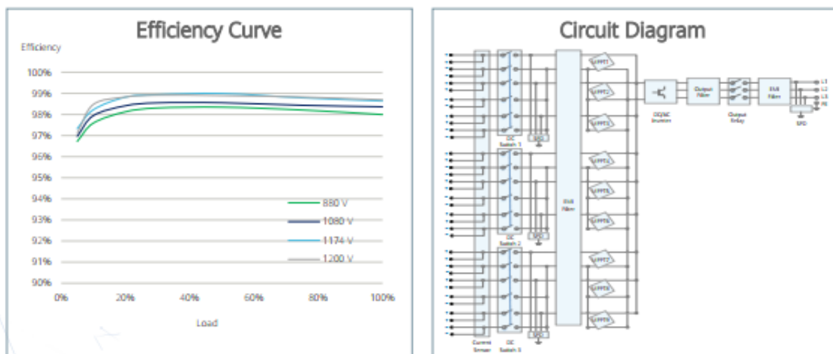
Fig. 13 - Dimensioni, specifiche tecniche e prestazionali dell'inverter
