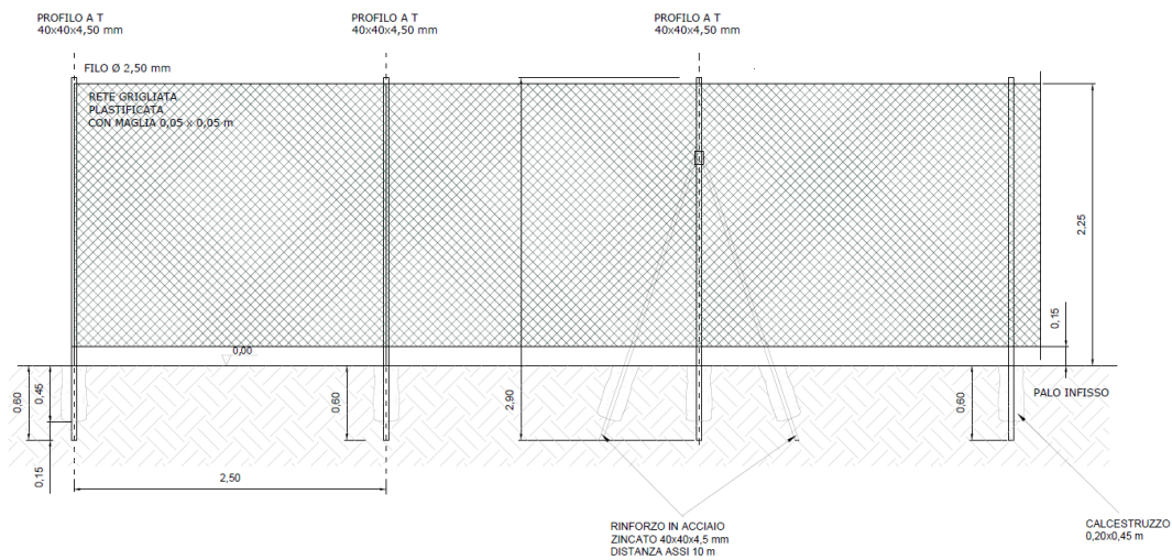
Fig. 16 – Particolare della recinzione
