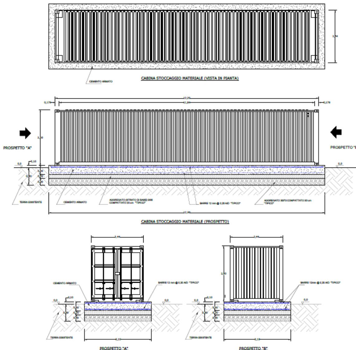
Fig. 14 - Cabina stoccaggio materiale
