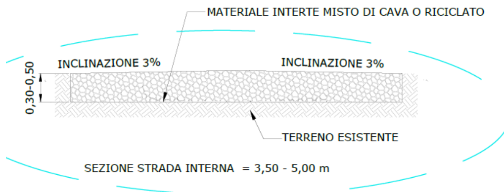
Fig. 18 – Sezione strada perimetrale
