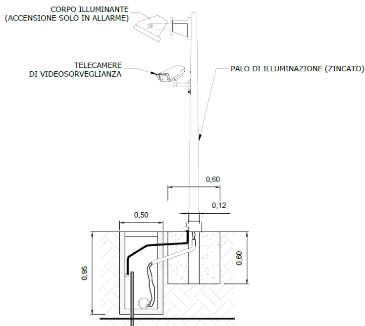
Fig. 2 – Sistema di illuminazione
