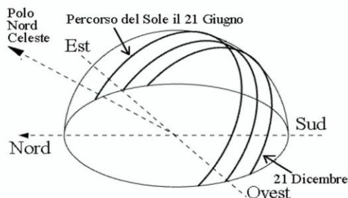
Fig. 3 - Movimento apparente del disco solare per un osservatore situato ad una latitudine nord attorno ai 45°. Per tutte le località situate tra il Tropic del Cancro e il Polo Nord Geografico il disco solare non raggiunge mai lo zenit.
