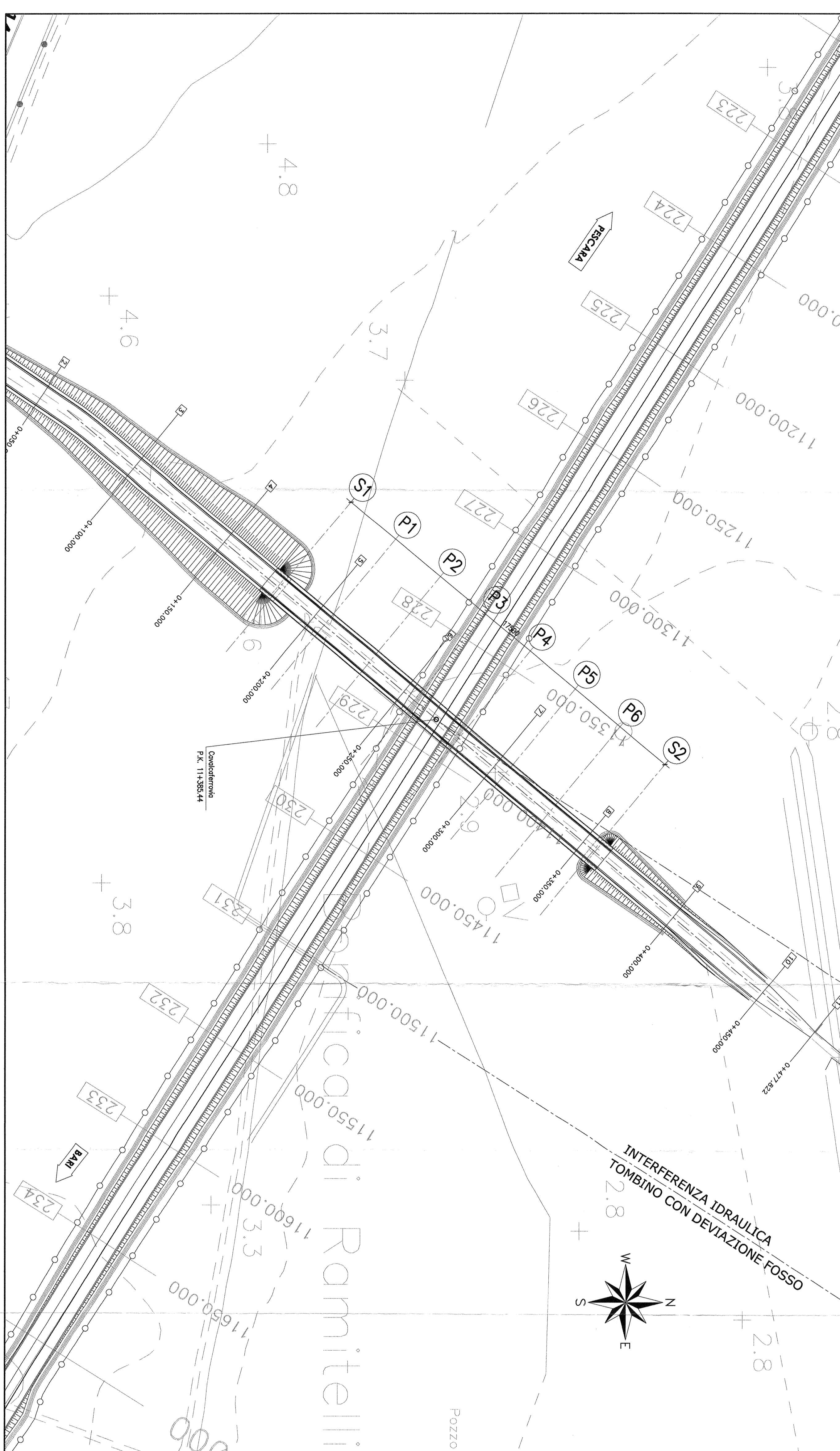
STRALCIO PLANIMETRICO "Cavalcavia progr.11+385.44" -Scala 1:1000
