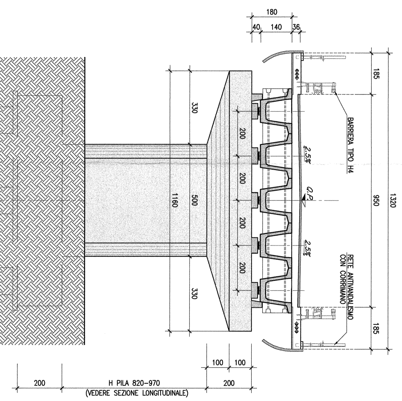
SEZIONE TRASVERSALE TIPO-Scala 1:100 (IN CAMPATA)
