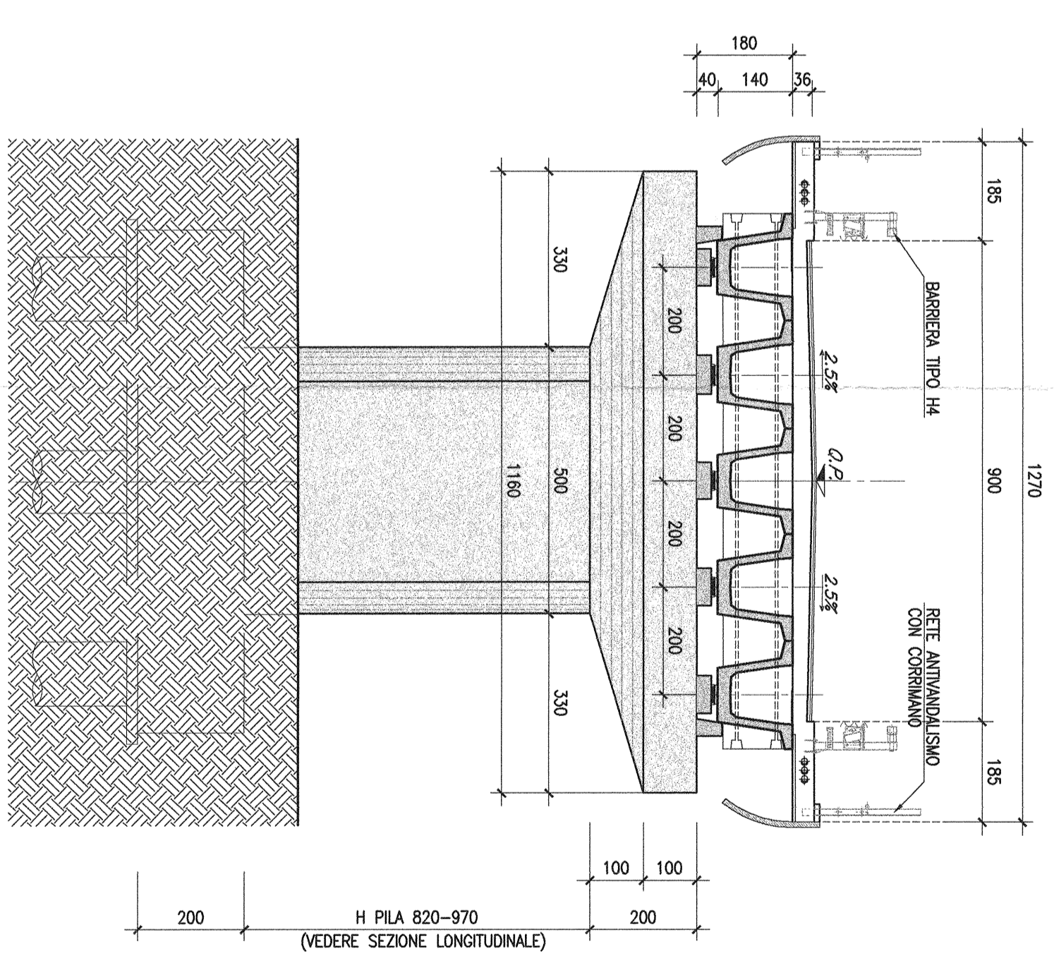
SEZIONE TRASVERSALE TIPO-Scala 1:100 (IN CAMPATA)
