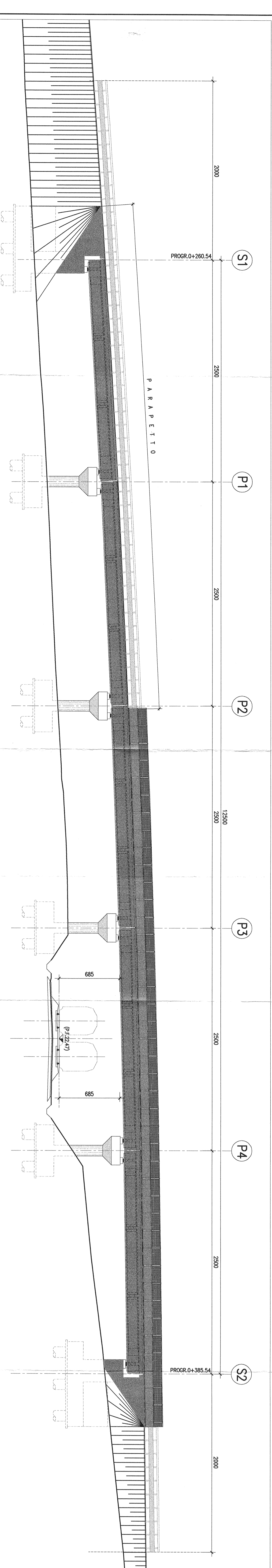
PROSPETTO "Cavalcavia progr.20+244" -Scala 1:200
