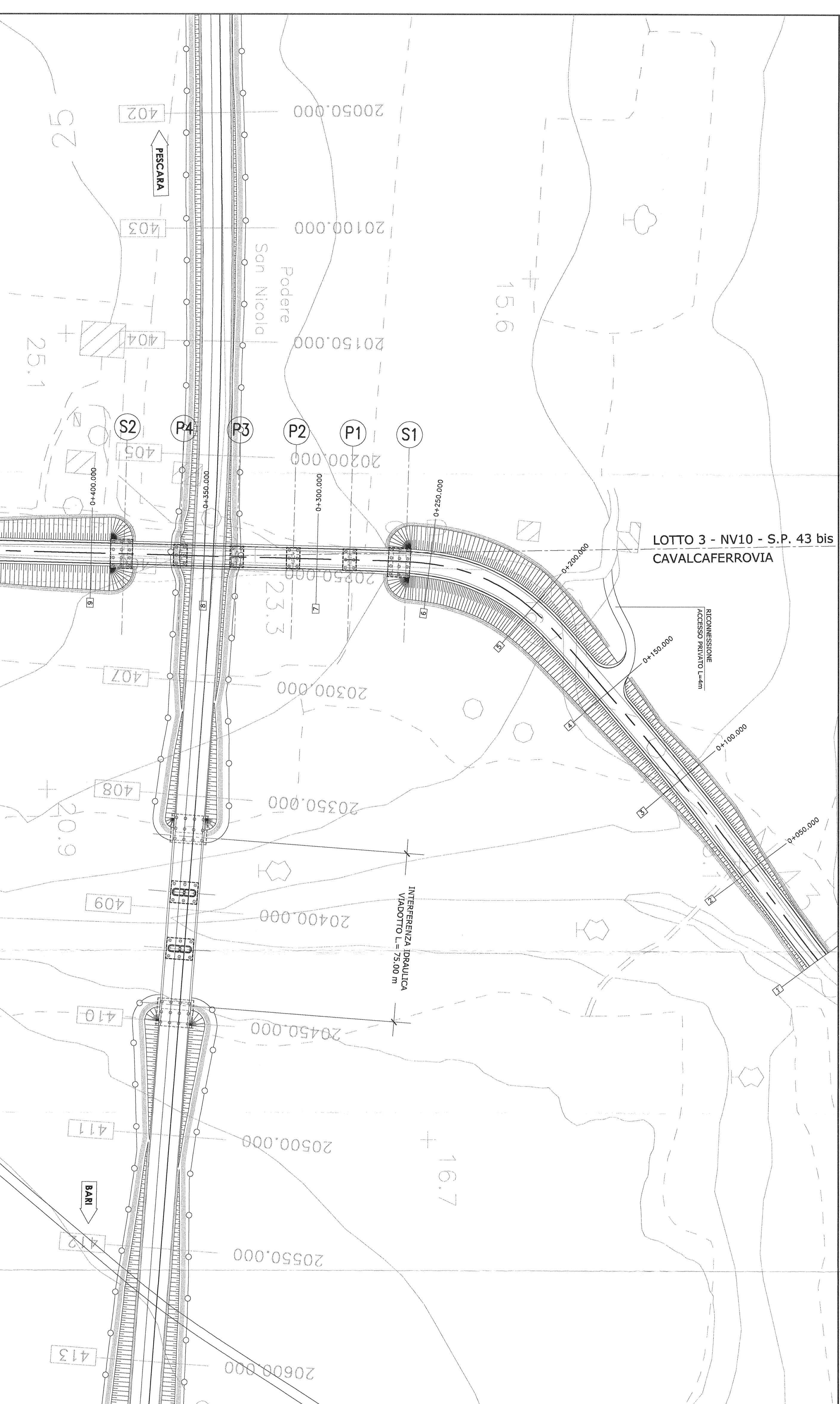
STRALCIO PLANIMETRICO "Cavalcavia progr.20+244" -Scala 1:1000
