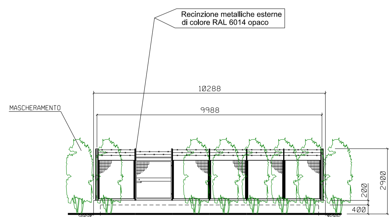
PROSPETTO A scala 1:100
