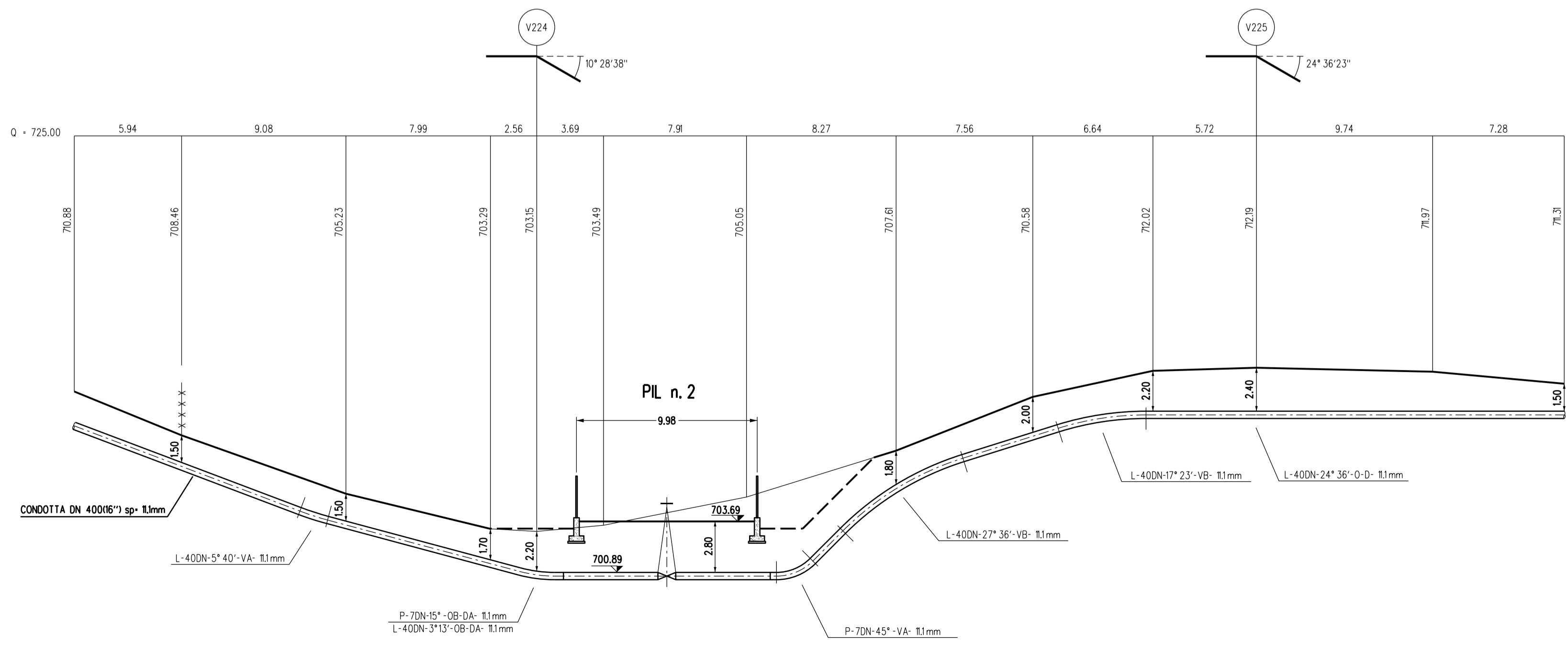
SEZIONE scala 1:200
