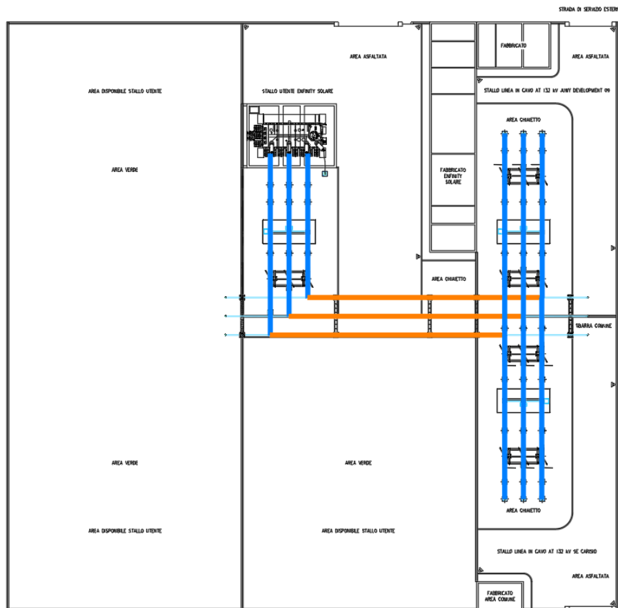
Figura 1 – Planimetria del punto di raccolta con individuazione degli elementi attivi
