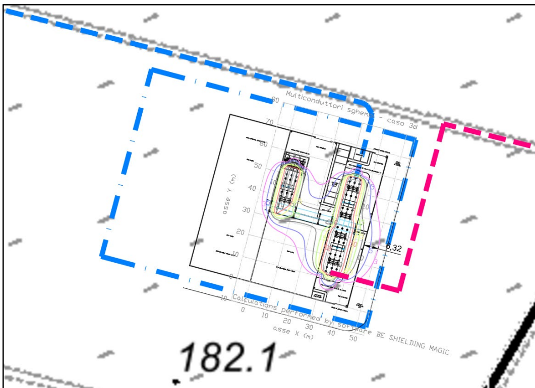
Figura 5 – Calcolo dei livelli di campo magnetico del punto di raccolta h=4 m dal suolo
