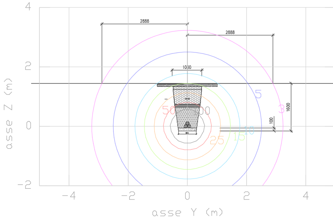
Figura 9 – Livelli di campo magnetico prodotti dal cavidotto AT interrato
