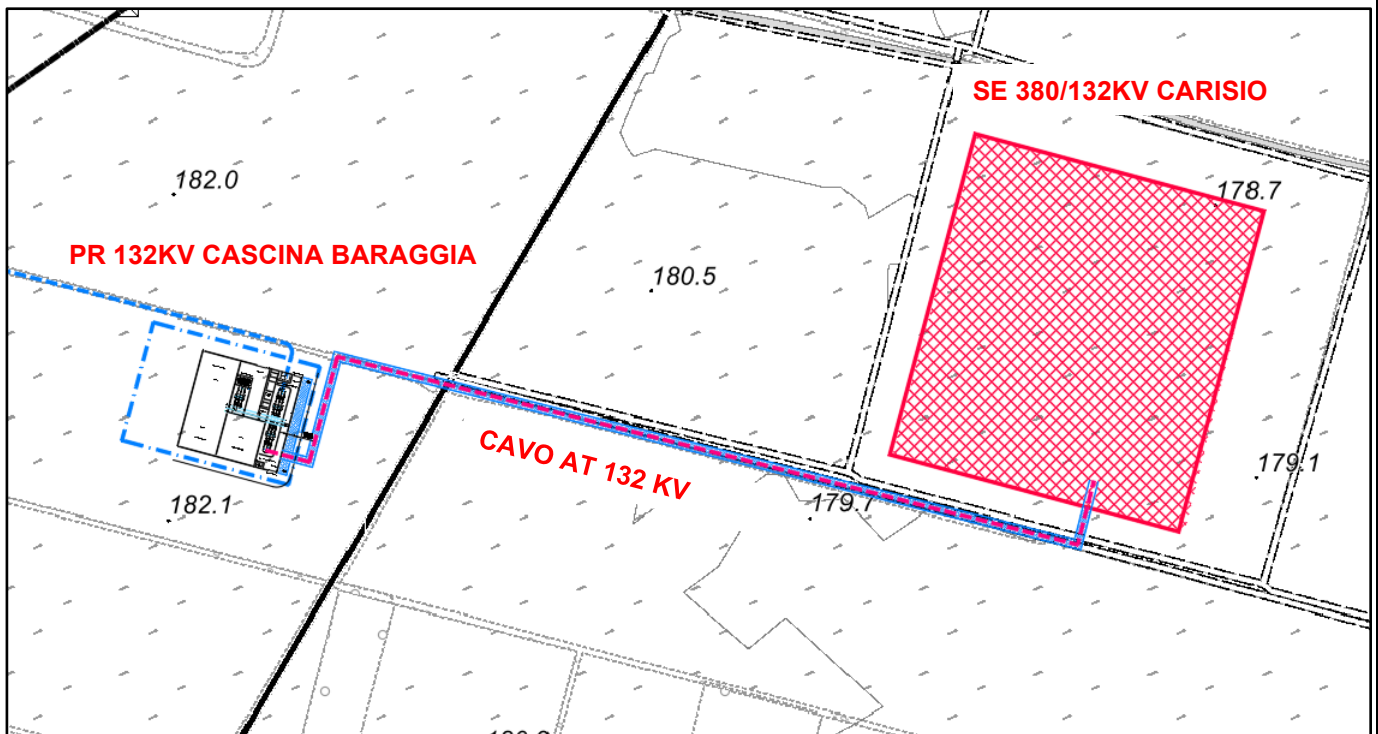
Figura 10 – Planimetria della Cabina Utente con indicazione della DPA
