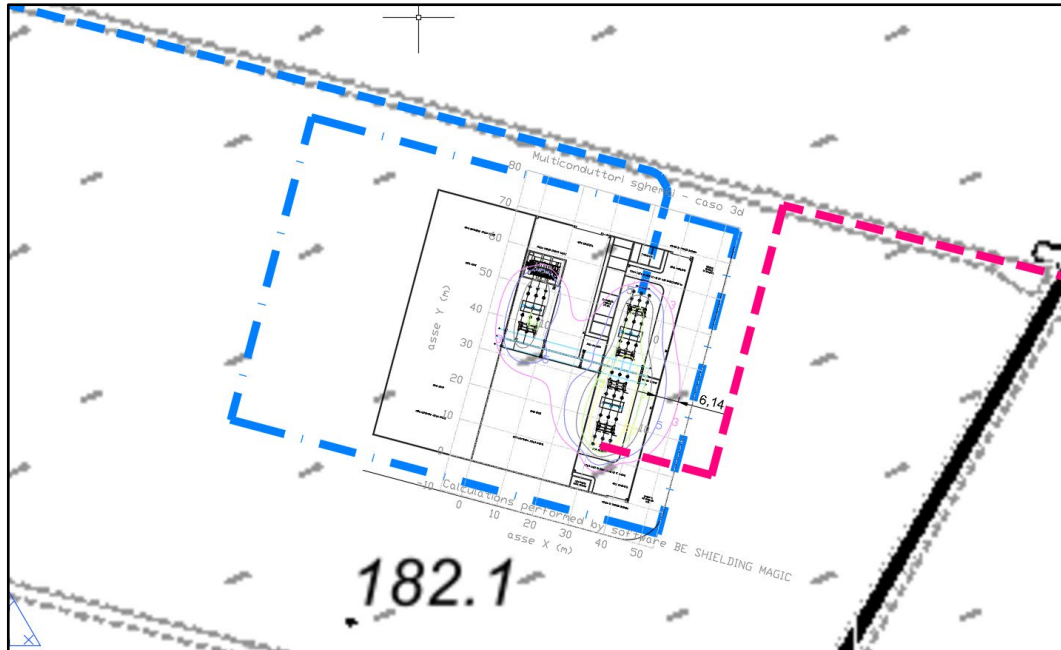
Figura 4 – Calcolo dei livelli di campo magnetico del punto di raccolta h=1m dal suolo
