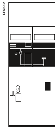
CRM Unità contattore 24 kV: 750 mm
