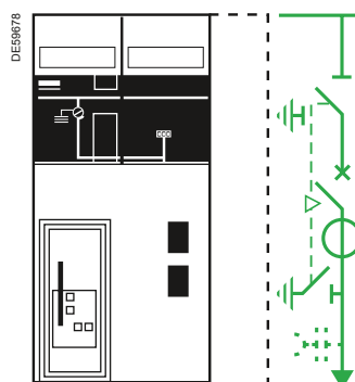
DM1-A Unità interruttore con sezionatore e partenza cavo 24 kV: 750 mm 36 kV: 1000 mm
