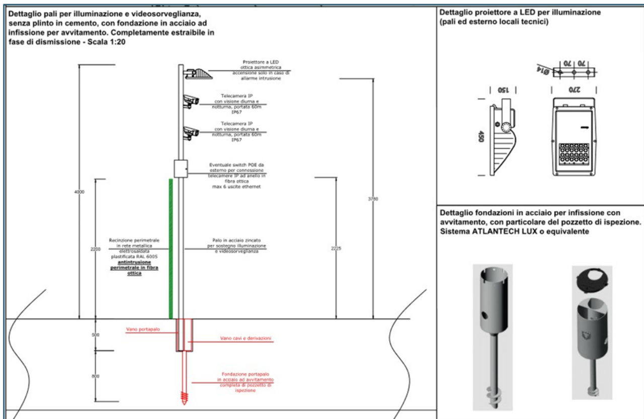
Figura 4. Esempio di infissione dei pali per telecamere TVCC e illuminazione
