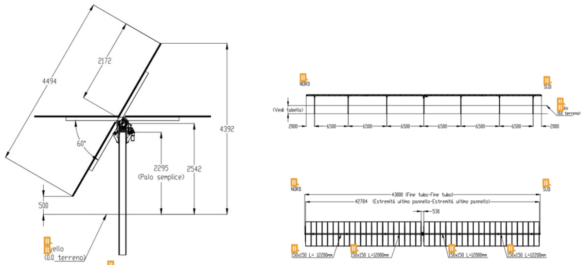
Figura 3. Struttura di supporto moduli
