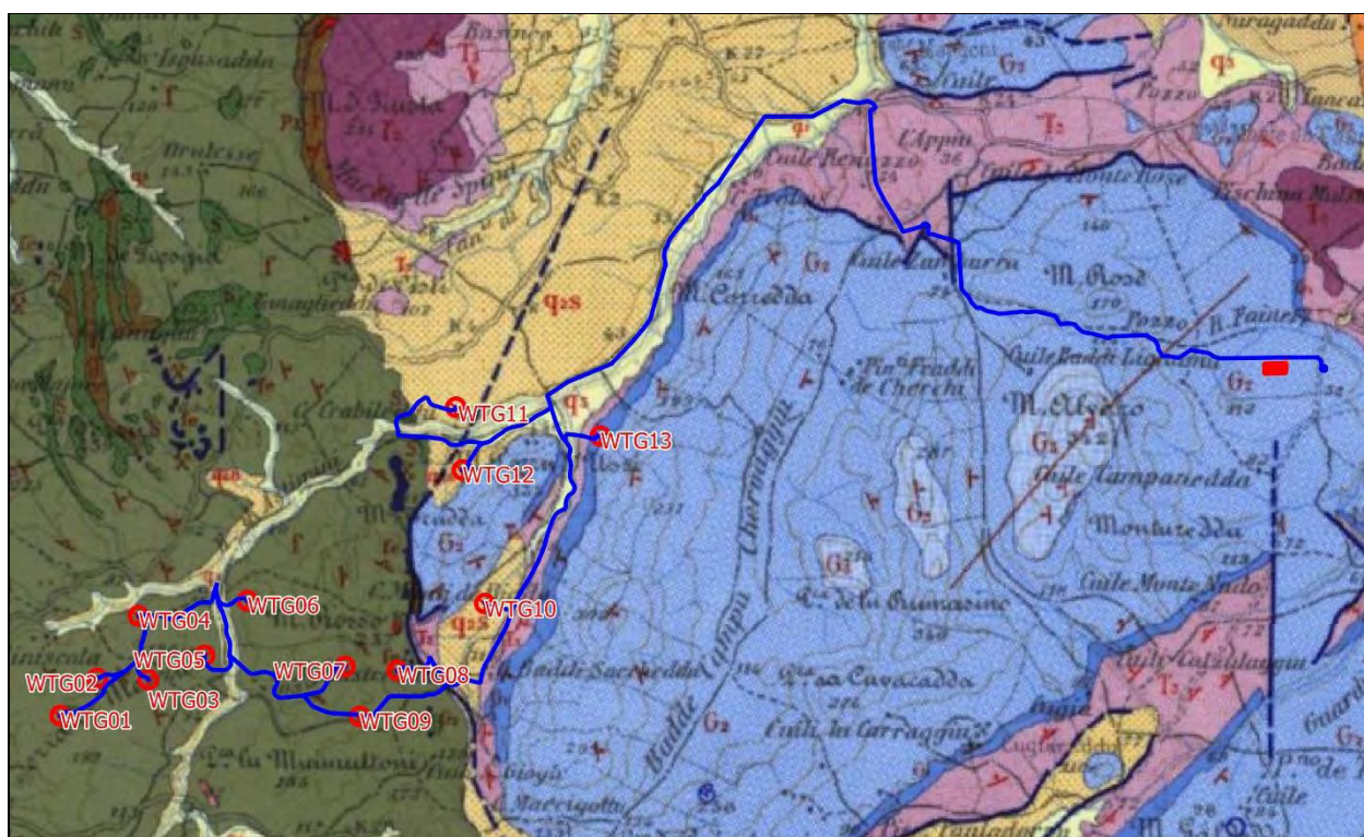
Fig. 02: Stralcio del Foglio 179 “Porto Torres” della Carta Geologica d’Italia, scala 1:100000 relativo al sito di progetto
