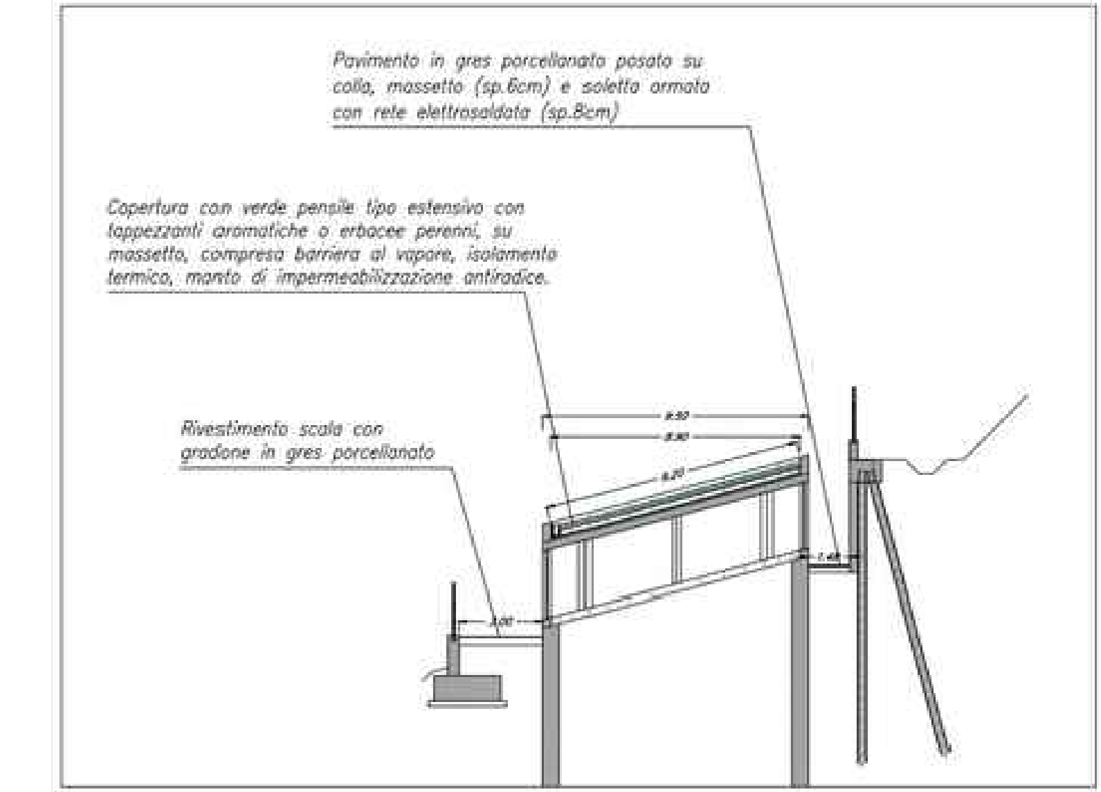
Pozzo di ventilazione 13+150km - Scala 1/200
