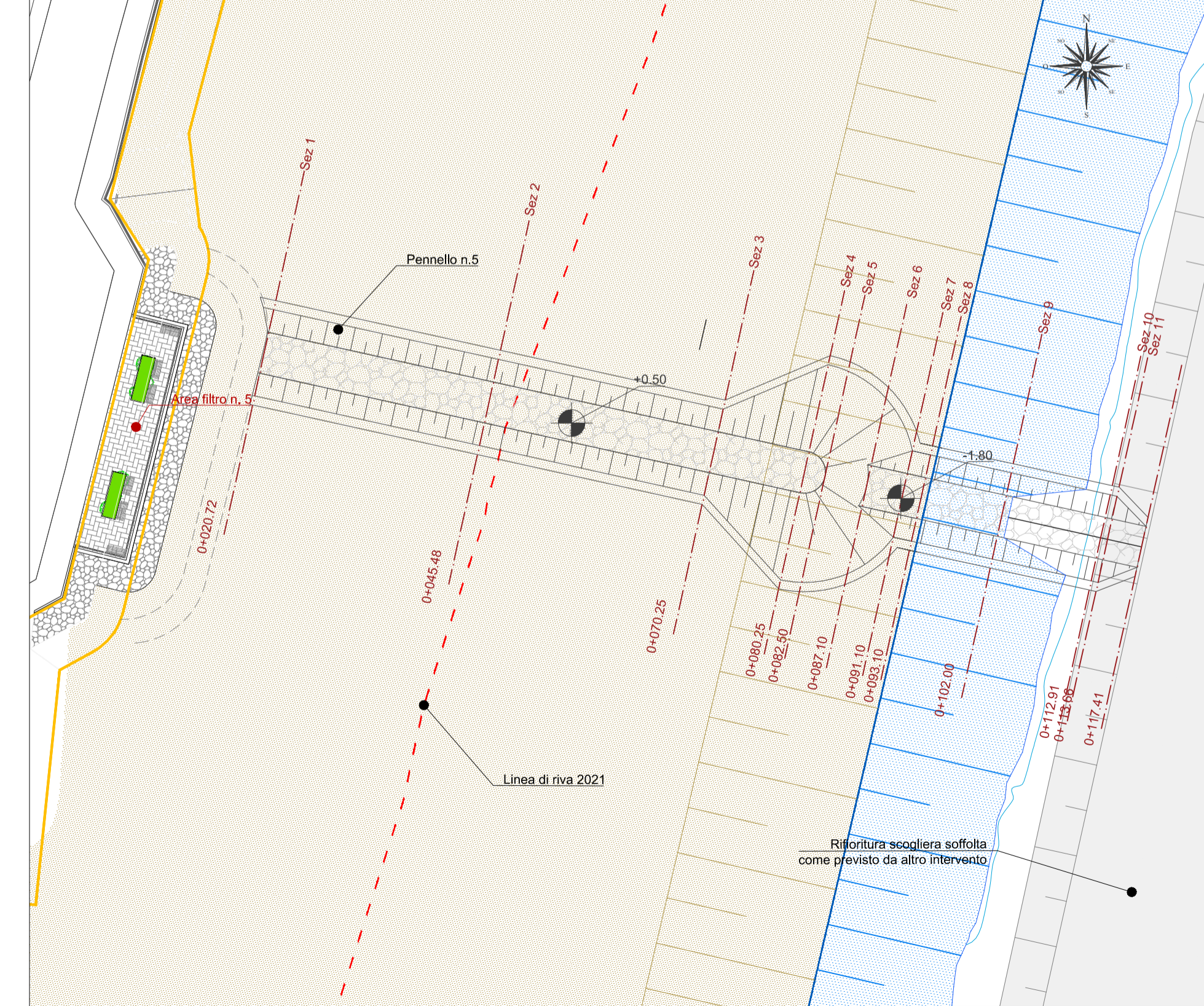
PLANIMETRIA (scala 1:500) - PENNELLO N.5
