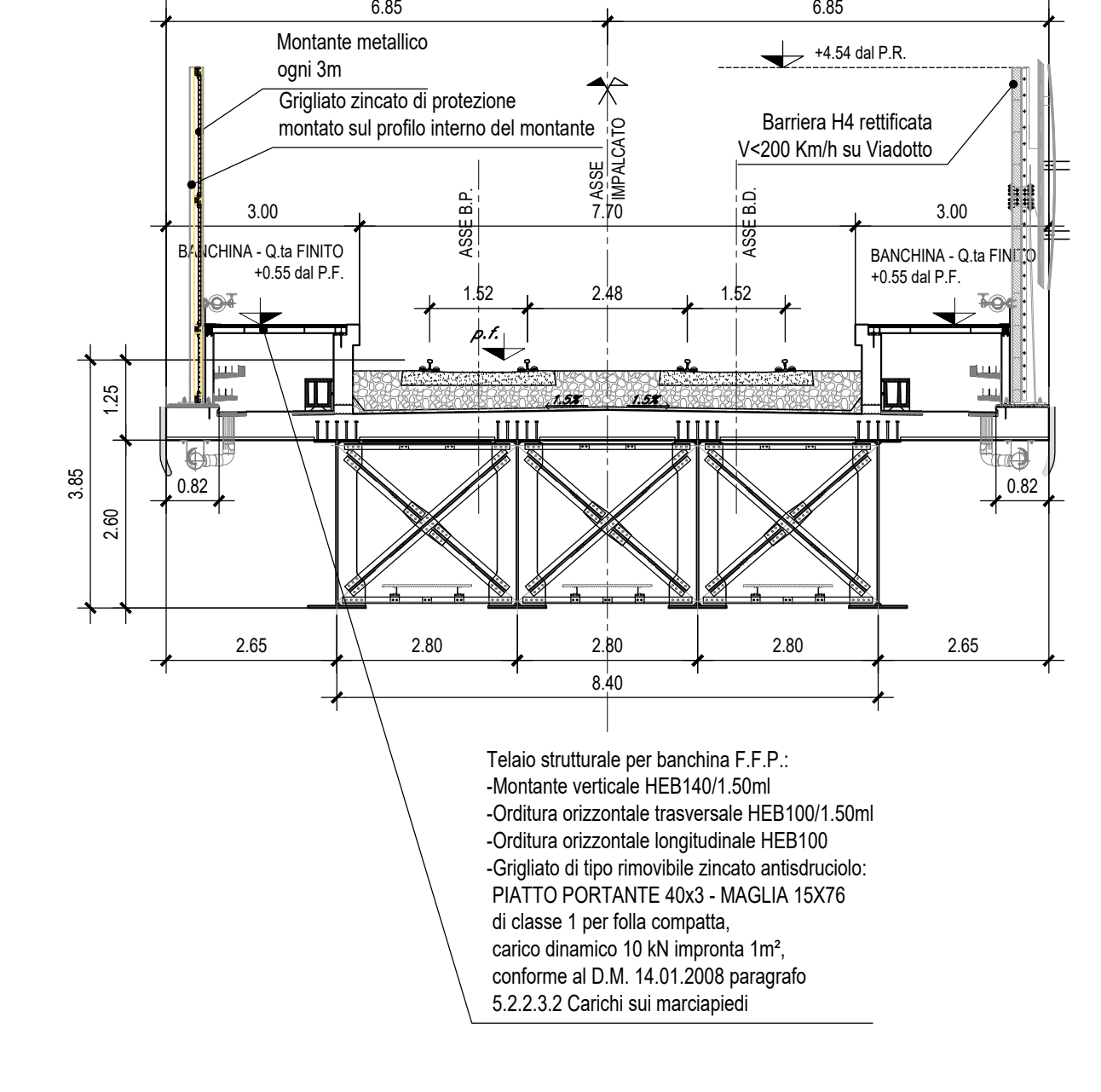
SEZIONE TIPO BANCHINA F.F.P.-Scala 1:100
