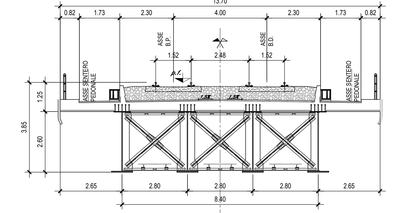
SEZIONE TIPO CORRENTE-Scala 1:100
