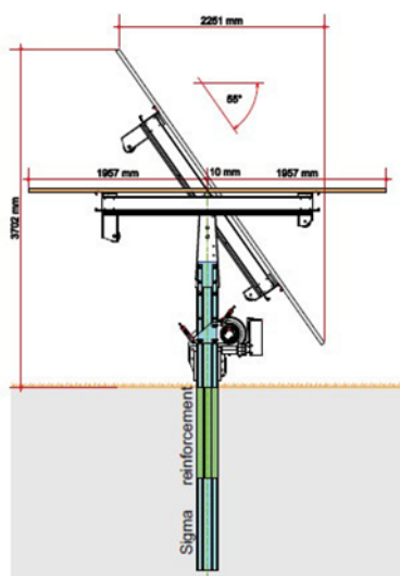
Figura 2 - struttura di sostegno dei pannelli fotovoltaici
