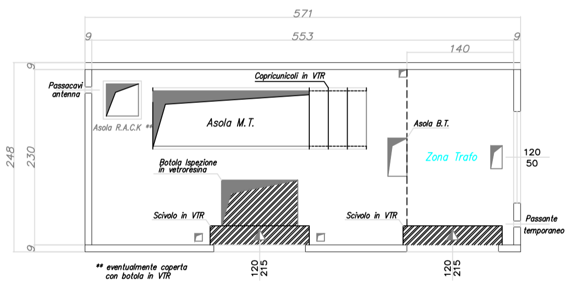
PIANTA
