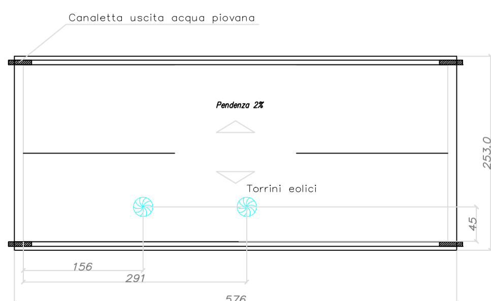
PIANTA COPERTURA
