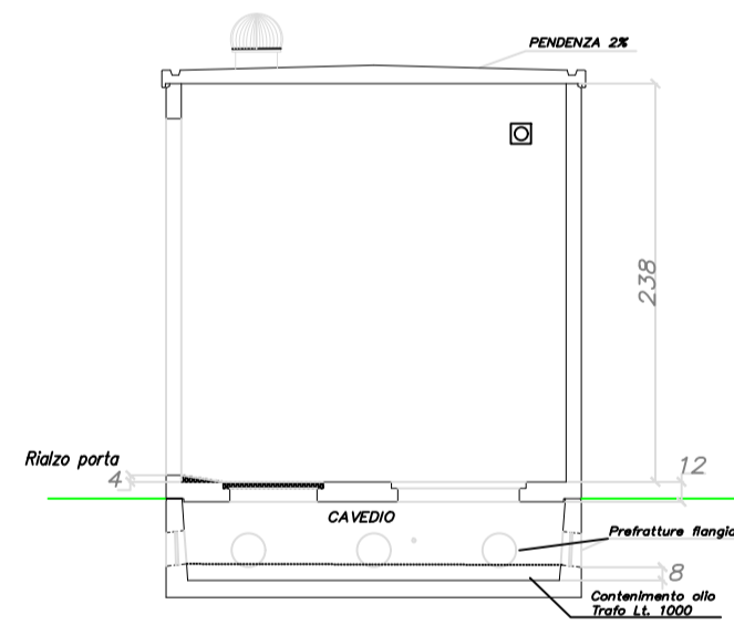
SEZ. TRASVERSALE
