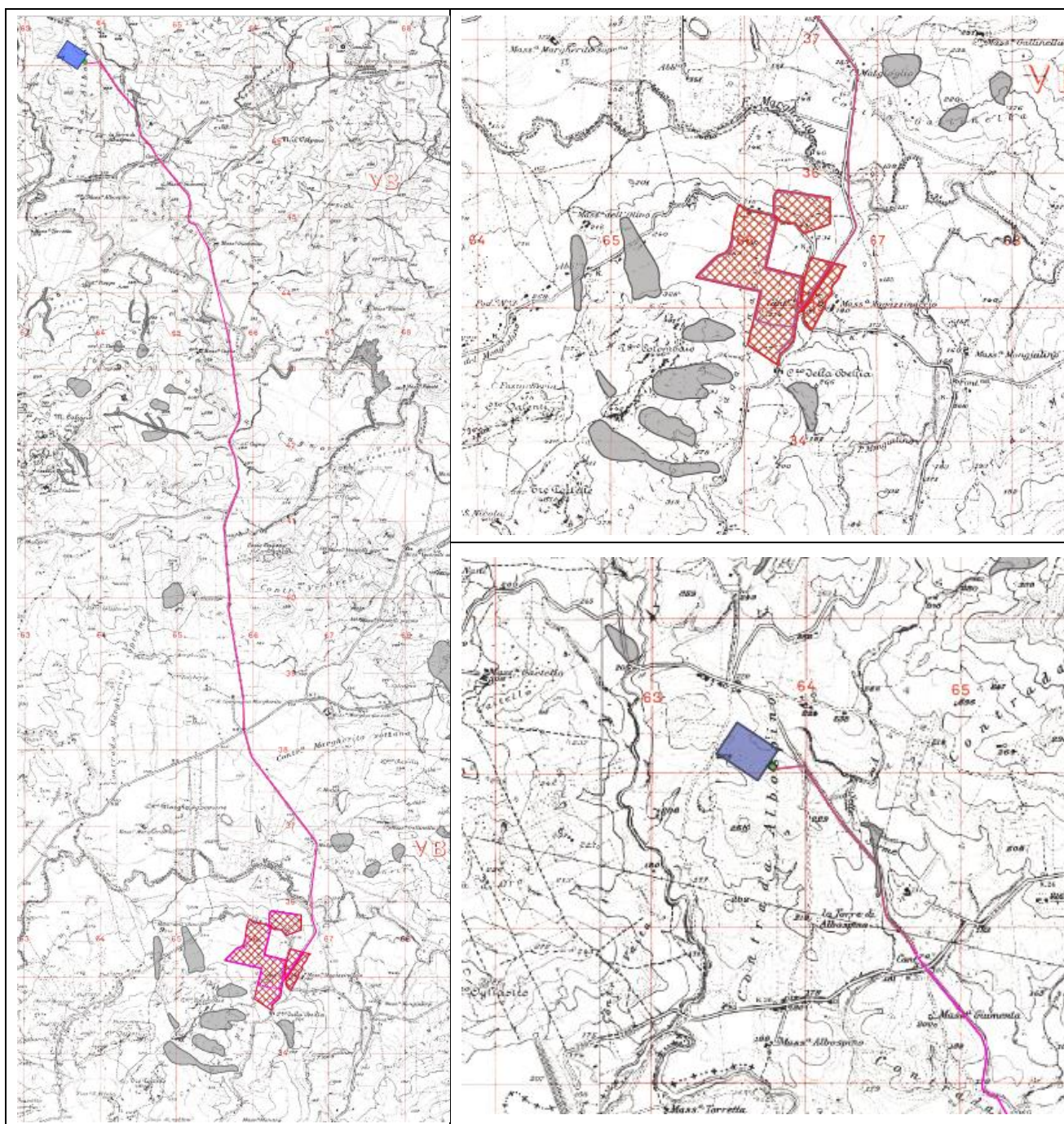
Fig. 03: PAI dell'AdB – Sede Sicilia, con ubicazione dell'area parco, del cavidotto e della Sottostazione Elettrica, con relativo quadro di unione
