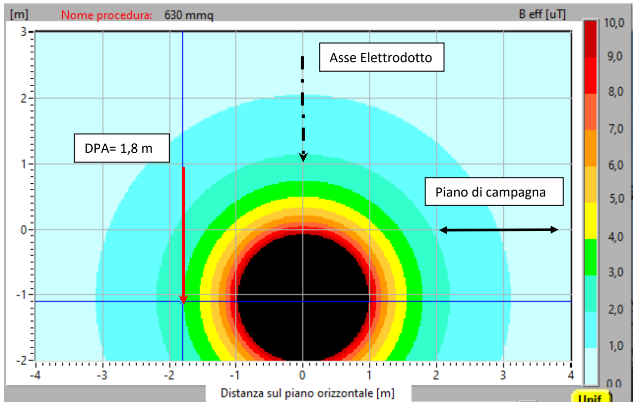
Figura 6 - Mappa verticale induzione magnetica (B) con indicazione della DPA – V=30 kV I = 703 A
