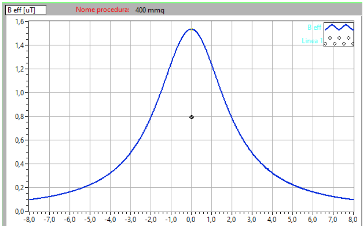
Figura 3 -Profilo laterale induzione magnetica (B) a 1 metro dal suolo –V=30 kV I = 543 A
