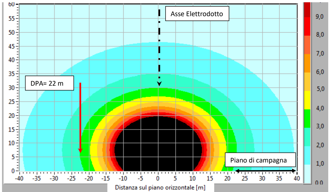
Fig. 18 Mappa verticale induzione magnetica (B) sbarre 150 kV
