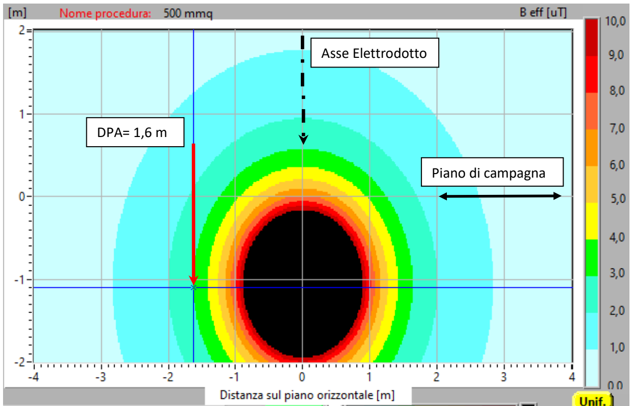
Figura 2 – Mappa verticale induzione magnetica (B) sezione tipo con indicazione della DPA – V=30 kV I = 618 A
