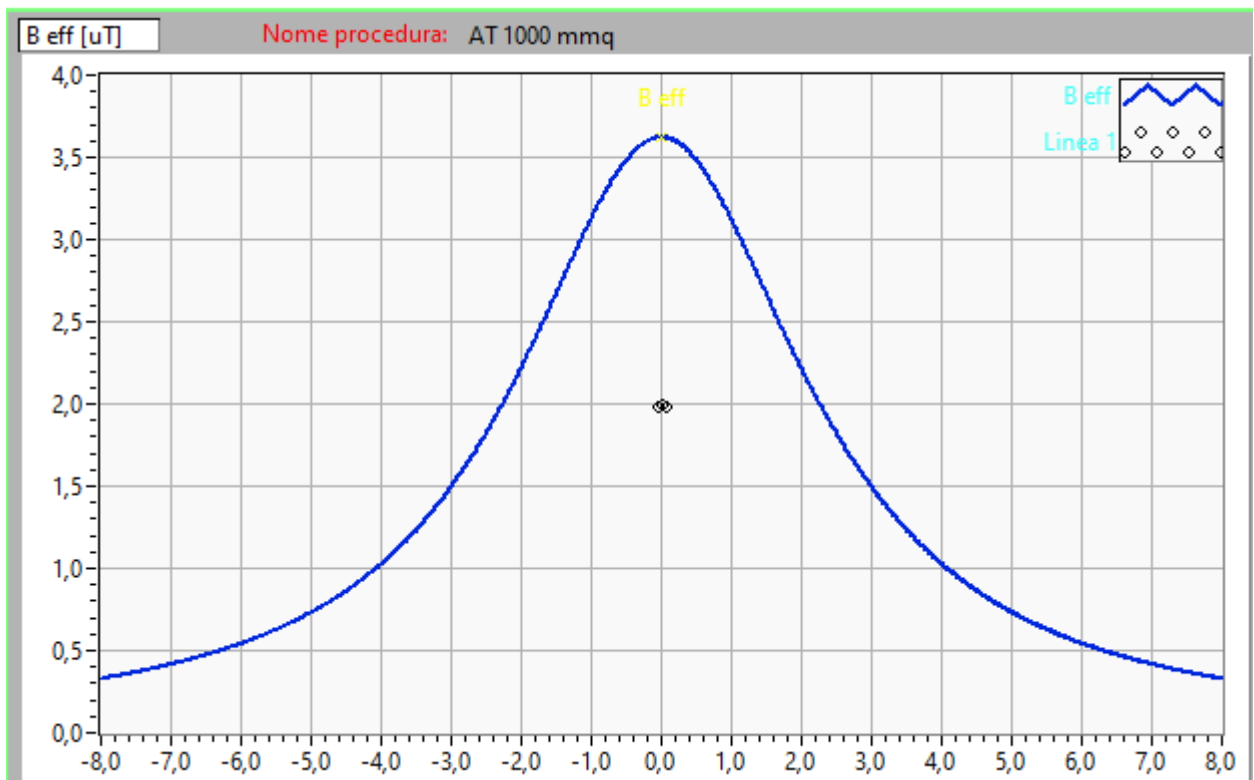
Fig. 13 Profilo laterale induzione magnetica (B) sezione tipo con indicazione della DPA - V=150 kV I = 910 A
