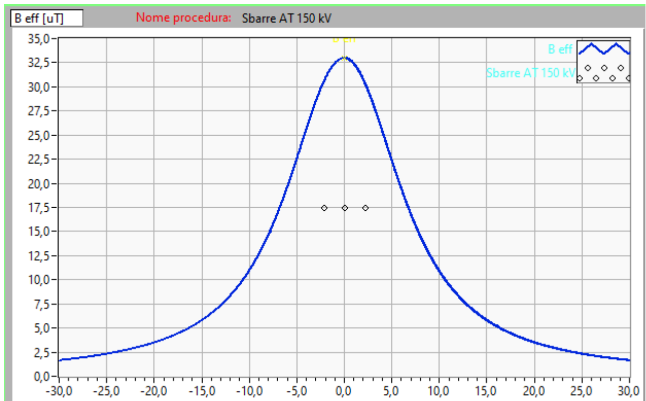
Fig. 17 Profilo laterale induzione magnetica (B) sbarre 150 kV
