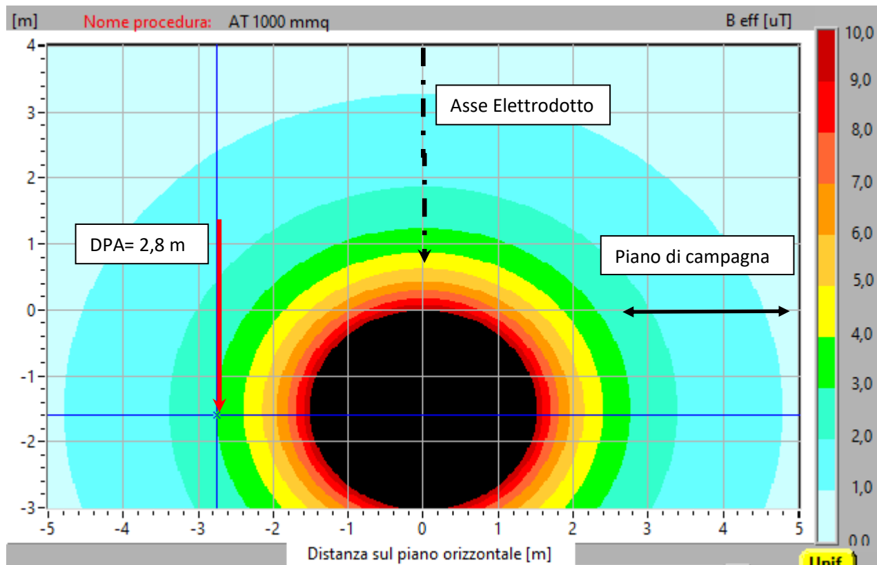
Fig. 14 Mappa verticale induzione magnetica (B) sezione tipo con indicazione della DPA - V=150 kV I = 910 A
