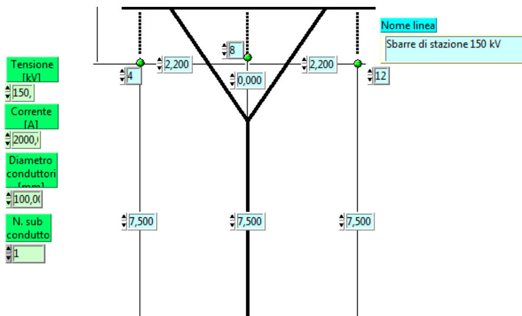
Fig. 15 Schema sezione sbarre 150 kV Stazione di trasformazione/condivisione 30/150 kV con caratteristiche geometriche e di carico
