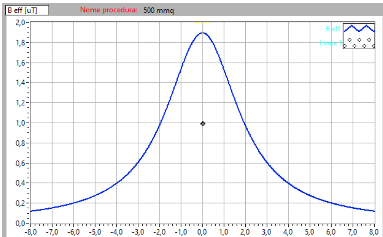
Figura 1 – Profilo laterale induzione magnetica (B) a 1 metro dal suolo – V=30 kV I = 618 A
