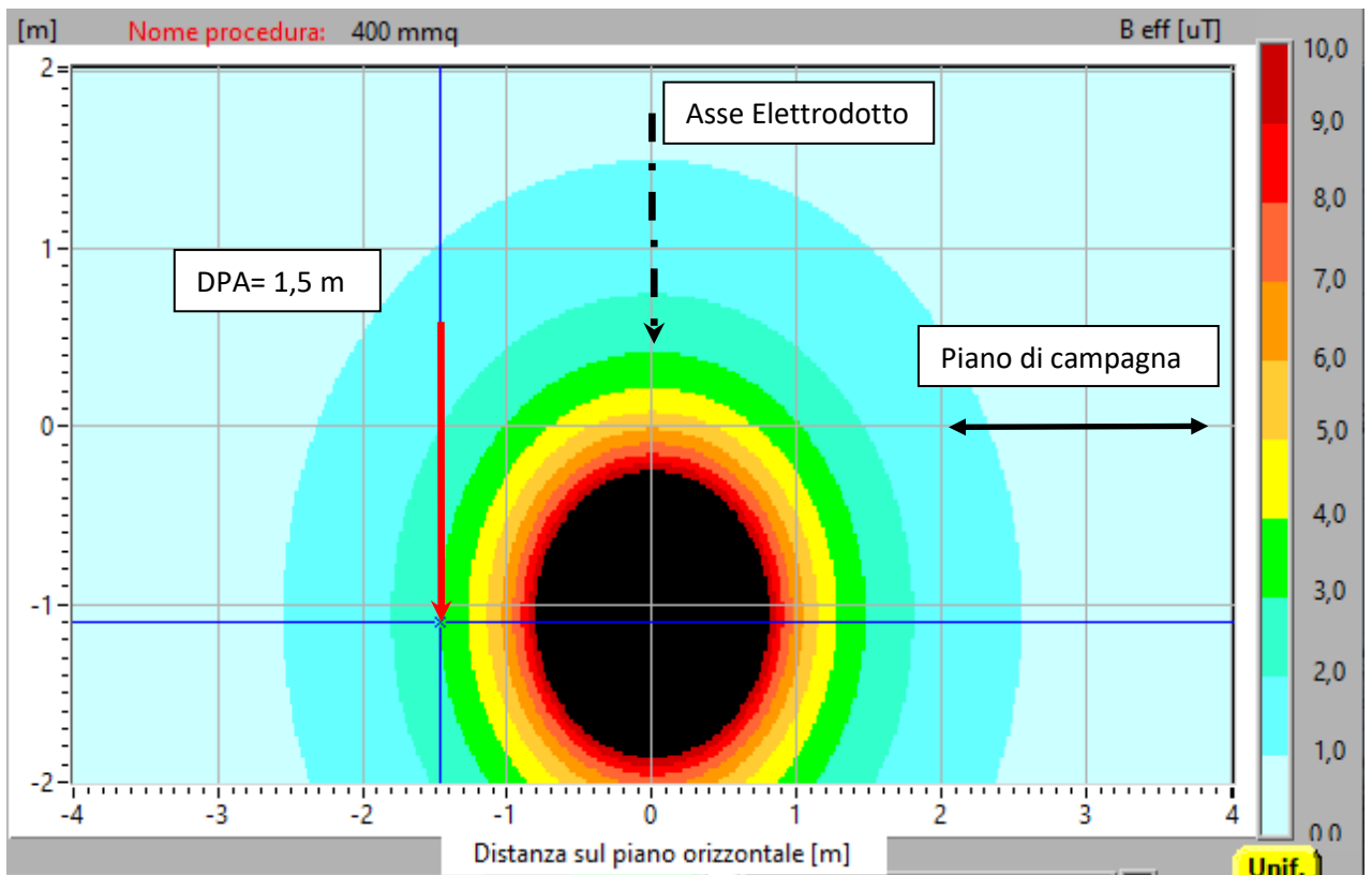
Figura 4 - Mappa verticale induzione magnetica (B) con indicazione della DPA – V=30 kV I = 543 A
