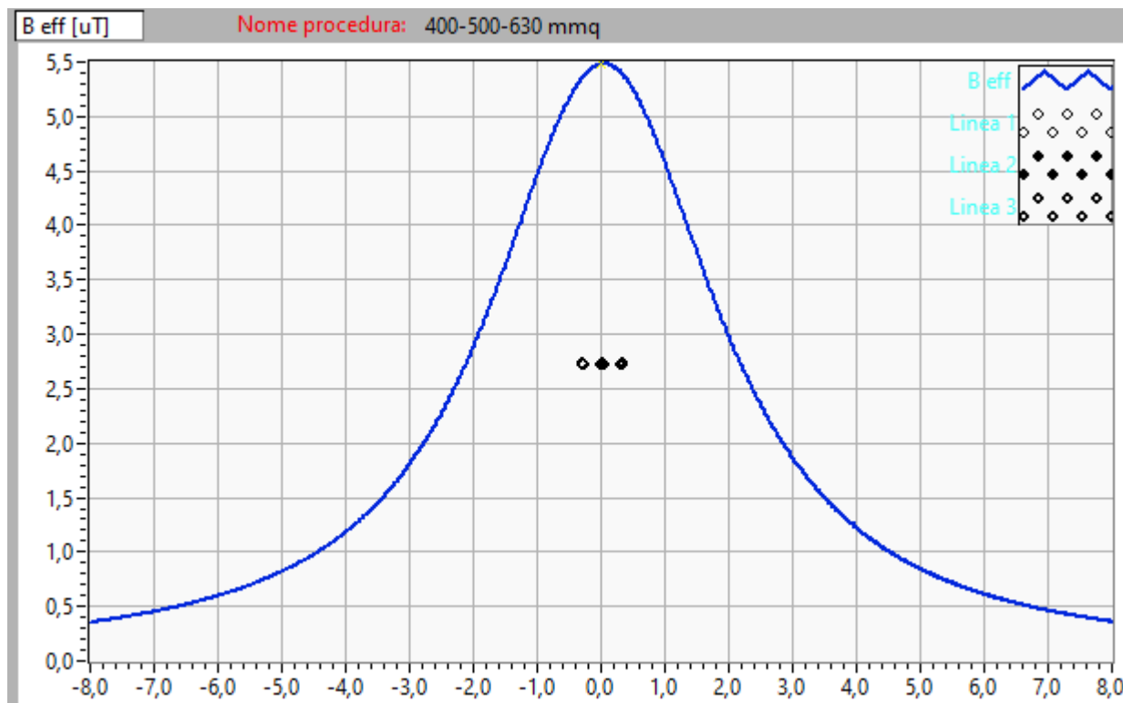
Figura 9 -Profilo laterale induzione magnetica (B) a 1 metro dal suolo -V=30 kV
