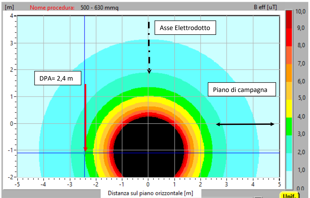
Figura 8 - Mappa verticale induzione magnetica (B) con indicazione della DPA - V=30 kV
