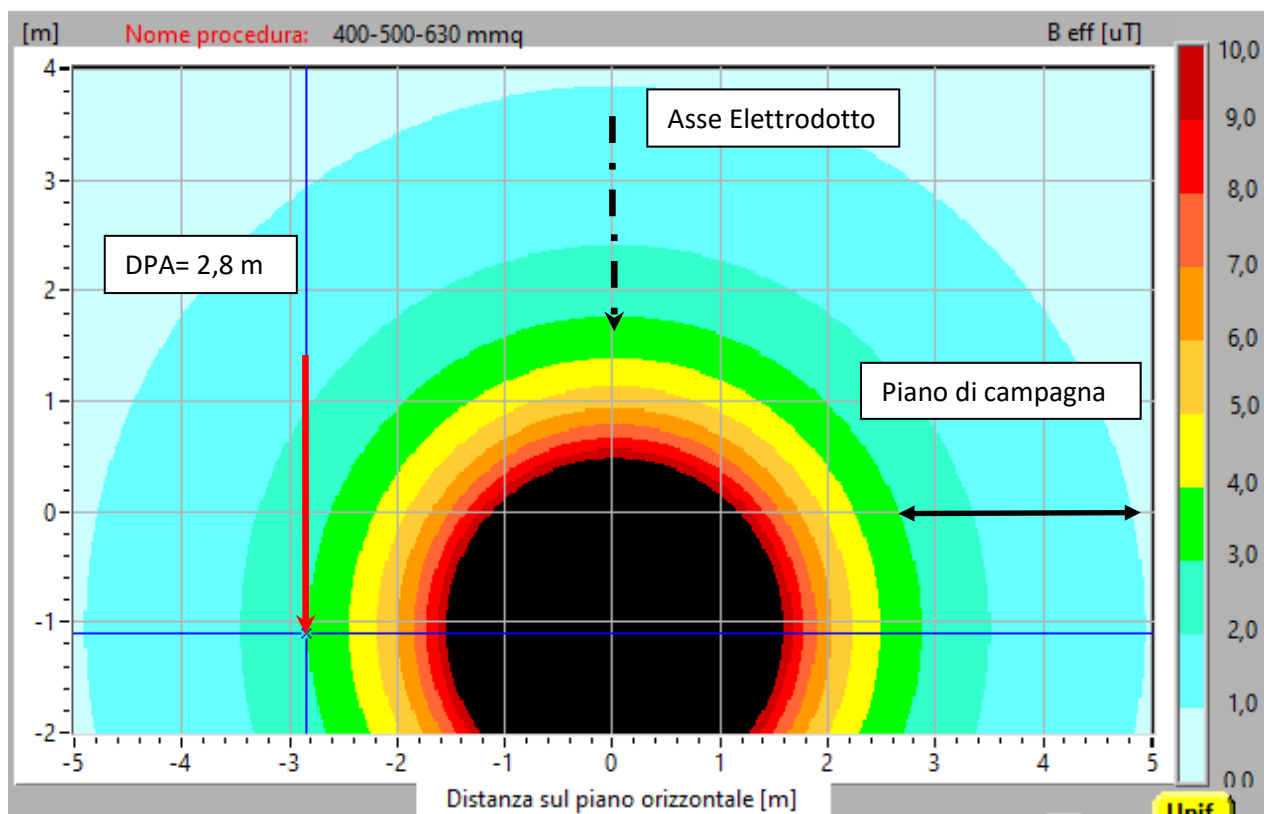
Figura 10 - Mapa verticale induzione magnetica (B) con indicazione della DPA – V=30 kV
