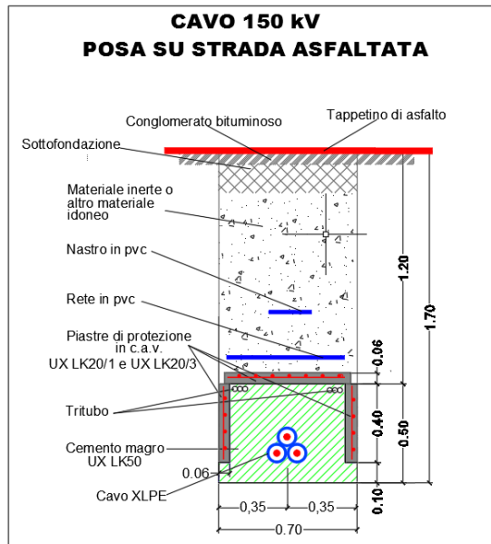
Figura 12: Posa cavo 150 kV “SE 30/150 kV – SE RTN Smistamento Escalaplano”
