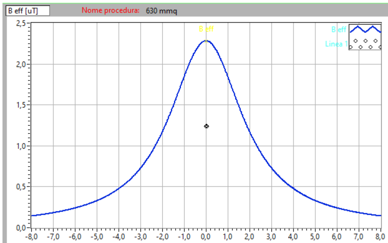
Figura 5 - Profilo laterale induzione magnetica (B) a 1 metro dal suolo -V=30 \text{ kV } I = 703 \text{ A}
