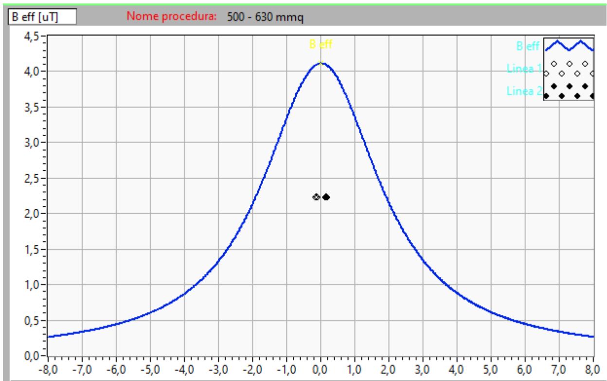
Figura 7 - Profilo laterale induzione magnetica (B) a 1 metro dal suolo -V=30 kV
