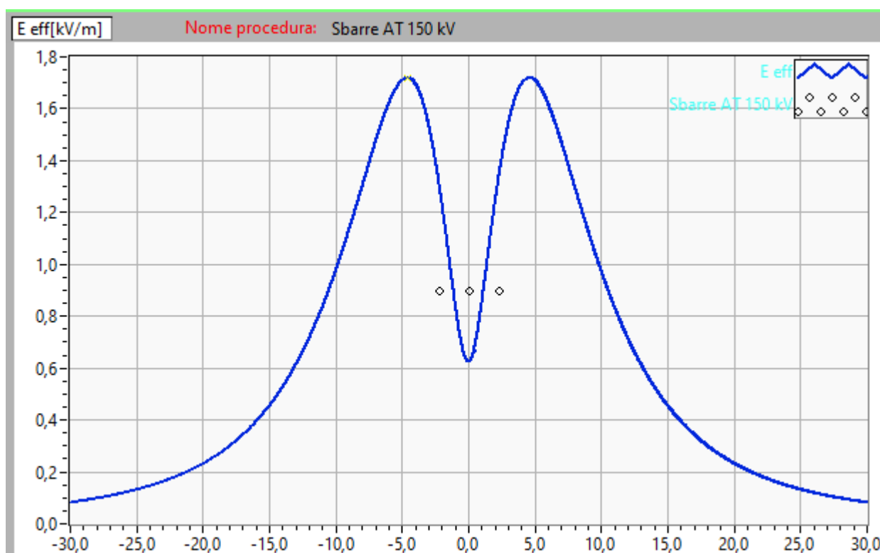
Fig. 16 Profilo laterale campo elettrico (E) sbarre 150 kV
