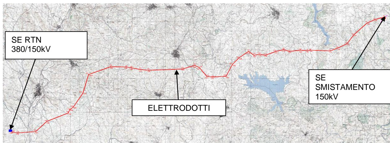
Fig.1 – Schema di connessione alla RTN della Futura SE di smistamento 150 kV con entra-esce della Linea 150 kV “Goni – Ulassai”
