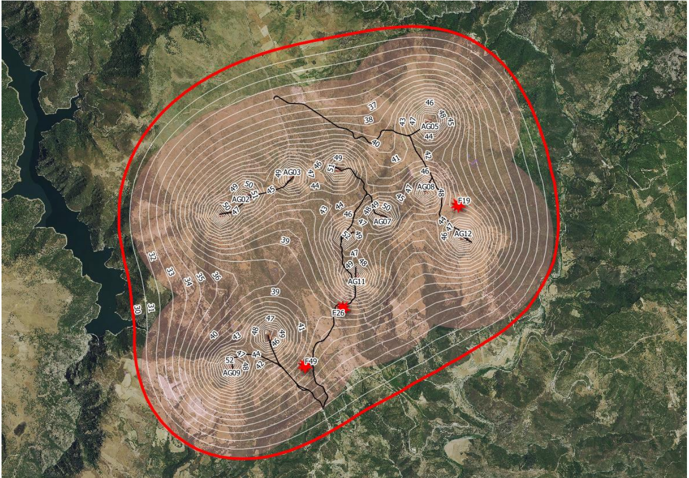
Figura 2.5 – Campo sonoro generato dall'impianto. In rosso l'isofonica dei 30 dBA, attestata ad una distanza indicativa di 1.000 m dalle postazioni eoliche in progetto
