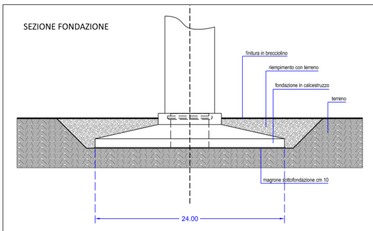
Figura 5.7 - Dettaglio sezione fondazione
