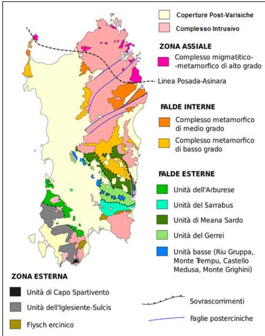
Figura 7.12 - Schema tettonico del Basamento varisico sardo
