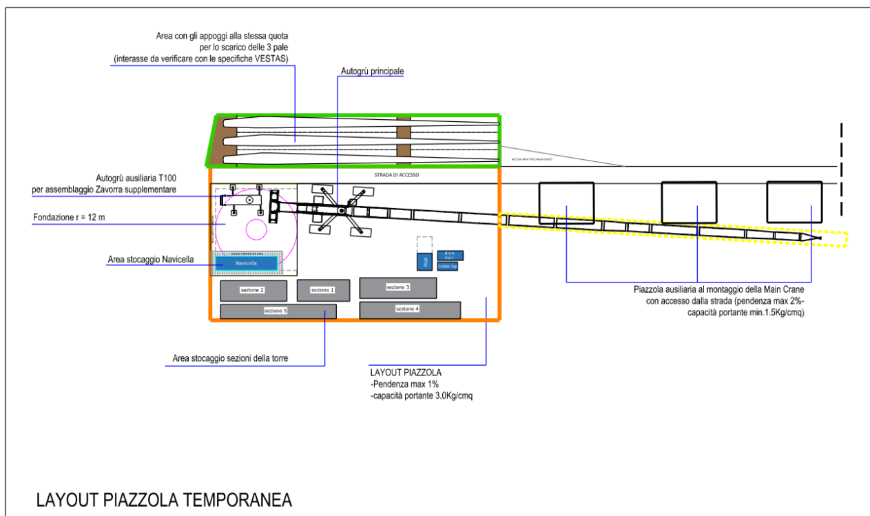
Figura 5.5 - Layout della piazzola temporanea
