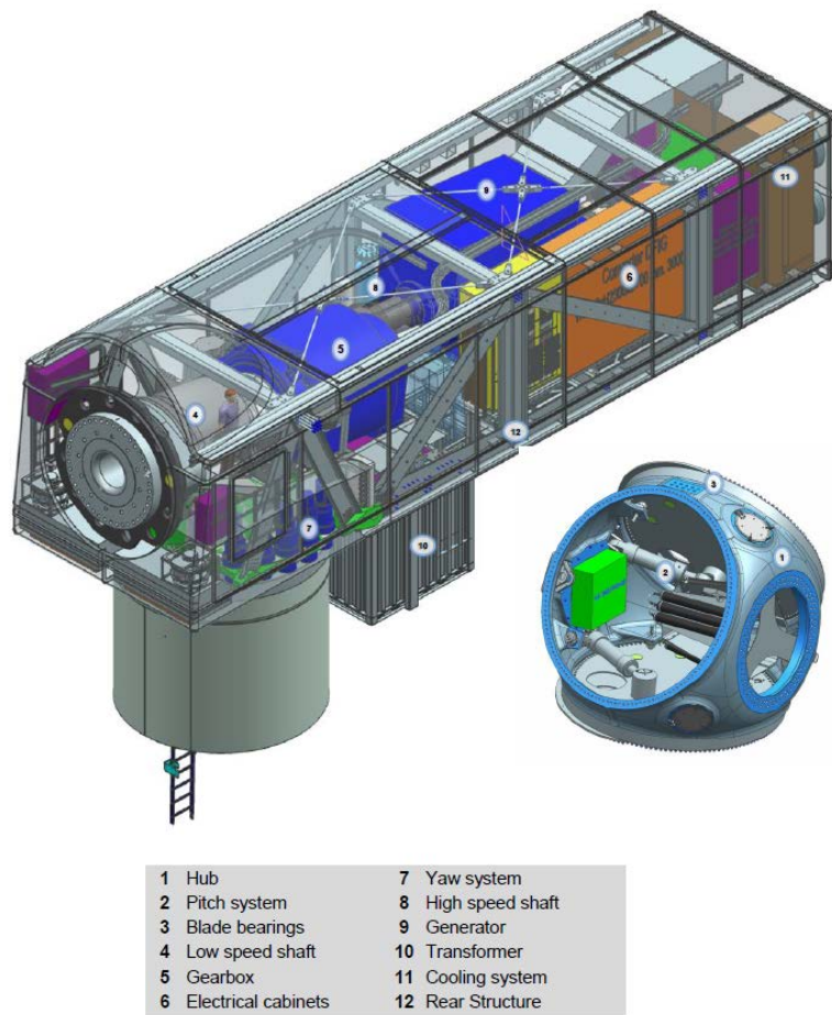
Figura 1 - Spaccato aerogeneratore tipo
