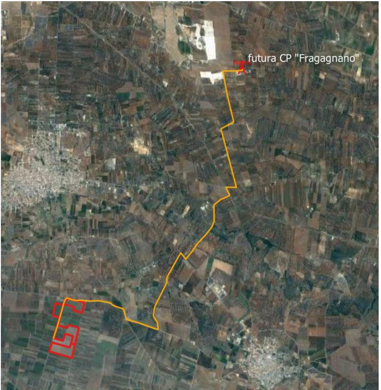
Figura 2 - Inquadramento dell'impianto FV e relative opere di connessione su ortofoto
