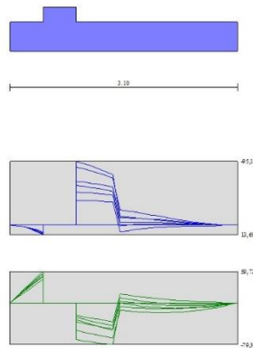
Figura 5: Involuppo CdS Fondazione.
