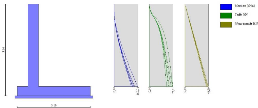
Figura 4: Inviluppo CdS paramento verticale.
