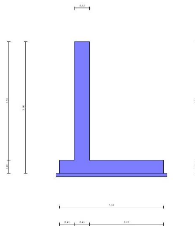
Figura 2: Geometria opera di sostegno.
