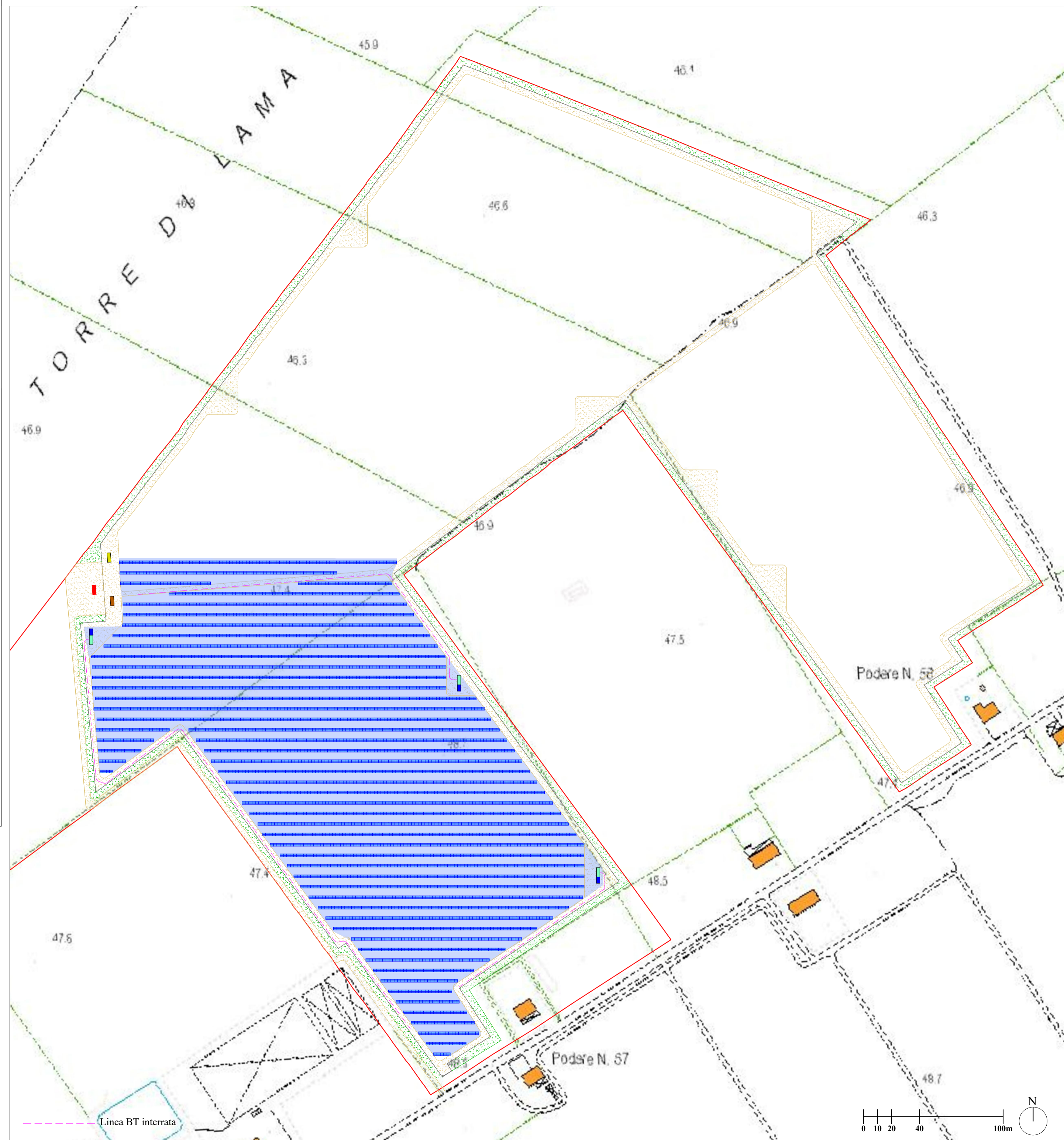
PLANIMETRIA TRACCIATO BT - TORRE DI LAMA 3 - IMPIANTO 1 - SCALA 1:2000
