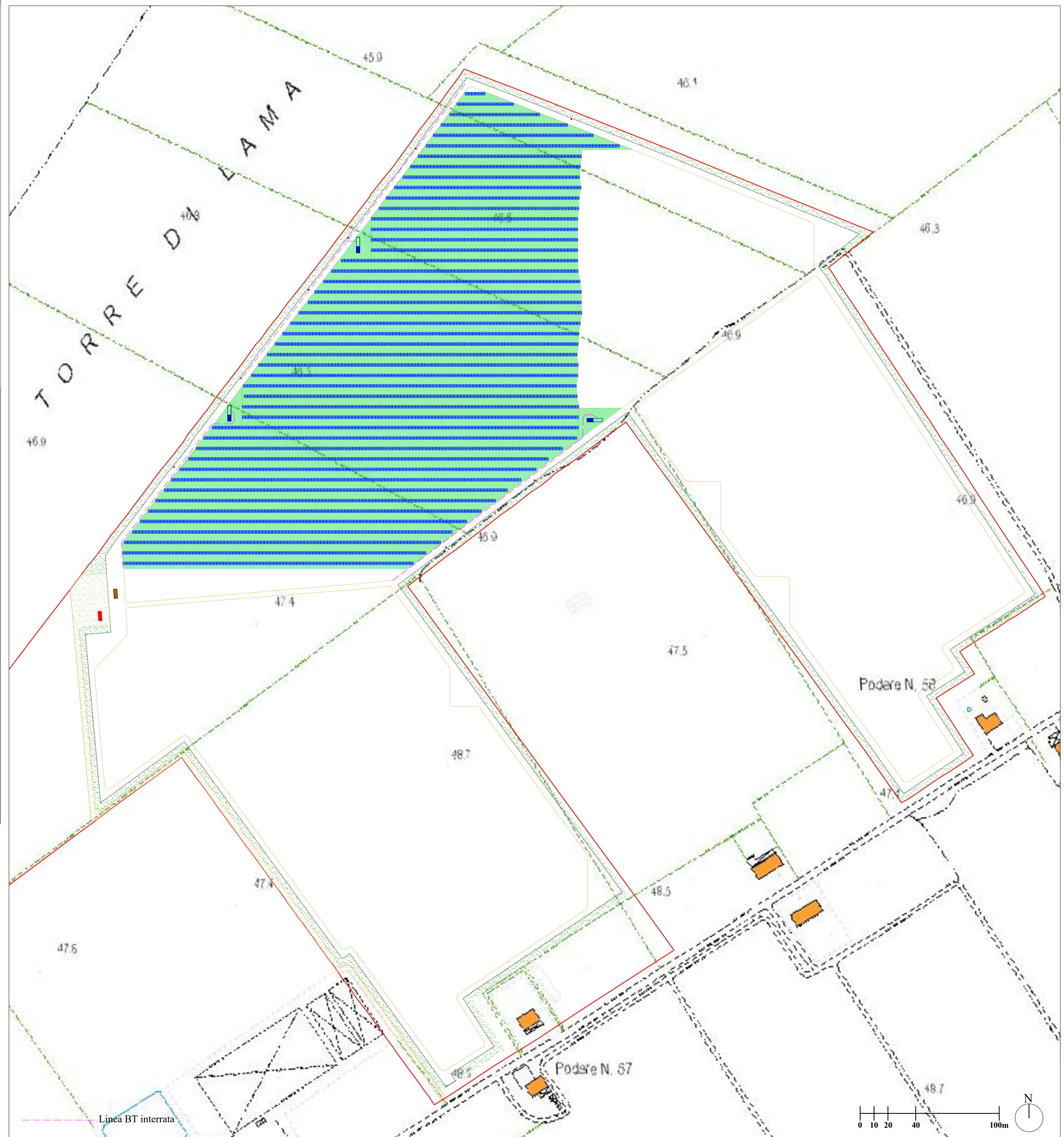
PLANIMETRIA TRACCIATO BT - TORRE DI LAMA 3 - IMPIANTO 2 - SCALA 1:2000
