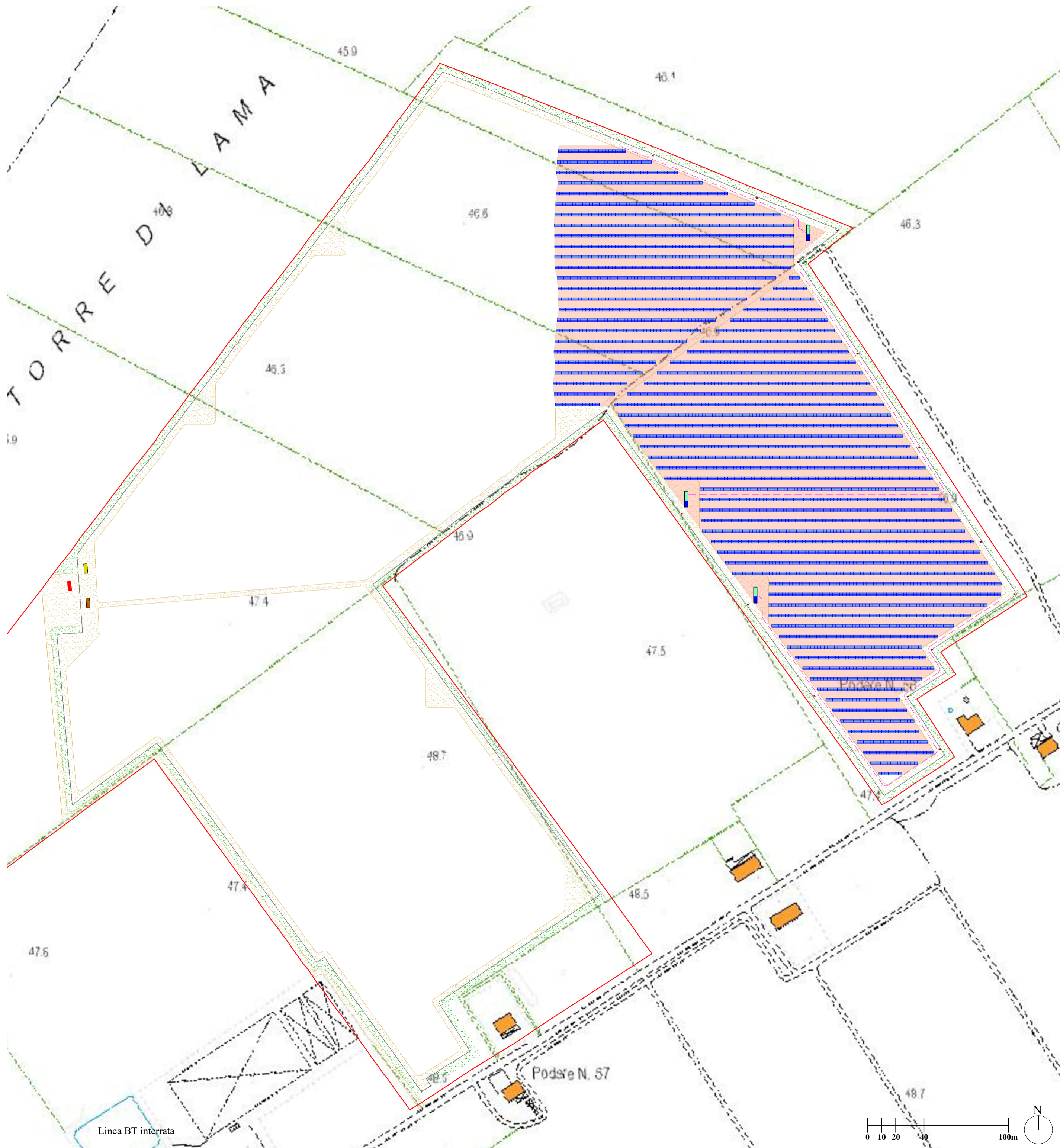
PLANIMETRIA TRACCIATO BT - TORRE DI LAMA 3 - IMPIANTO 3 - SCALA 1:2000
