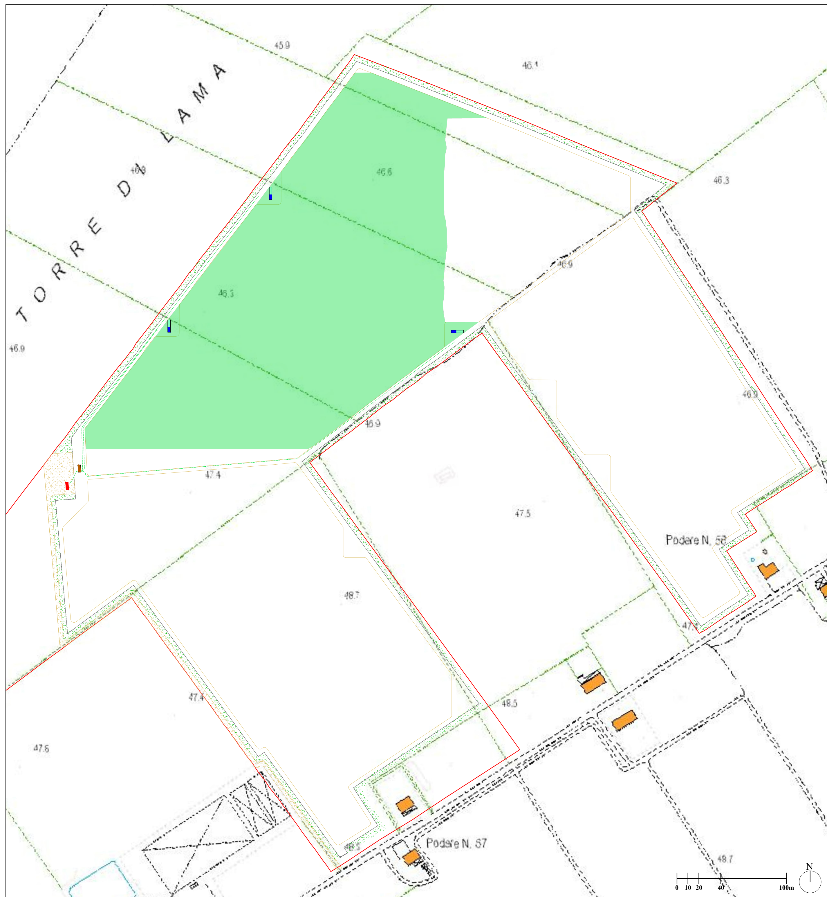
PLANIMETRIA TRACCIATO MT - TORRE DI LAMA 3 - IMPIANTO 2 - SCALA 1:2000
