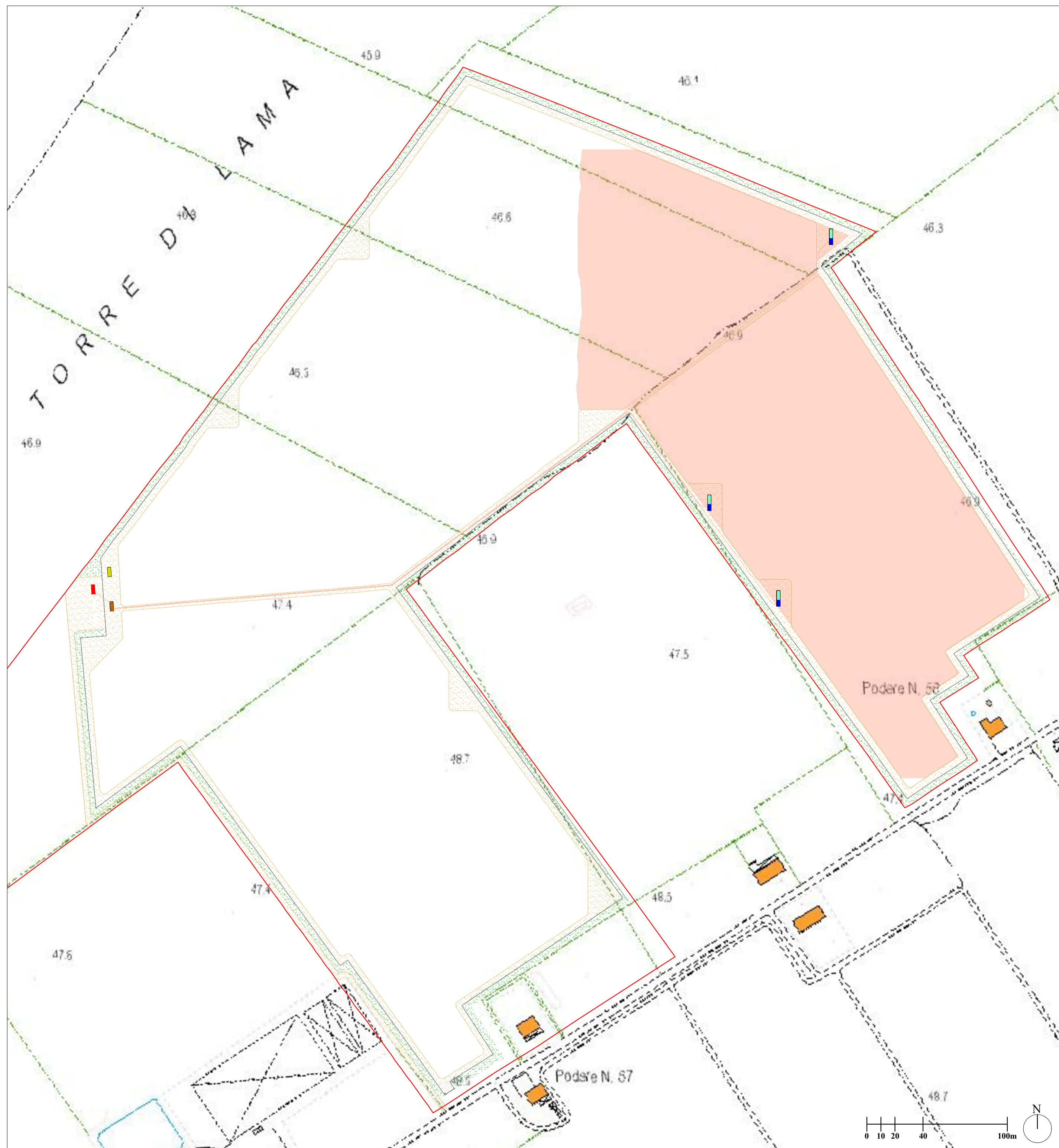
PLANIMETRIA TRACCIATO MT - TORRE DI LAMA 3 - IMPIANTO 3 - SCALA 1:2000
