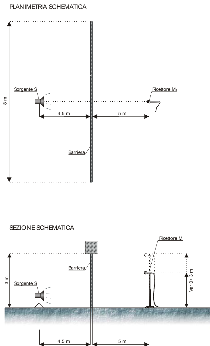
Figura F: schema della prova su elementi antidiffrittivi
